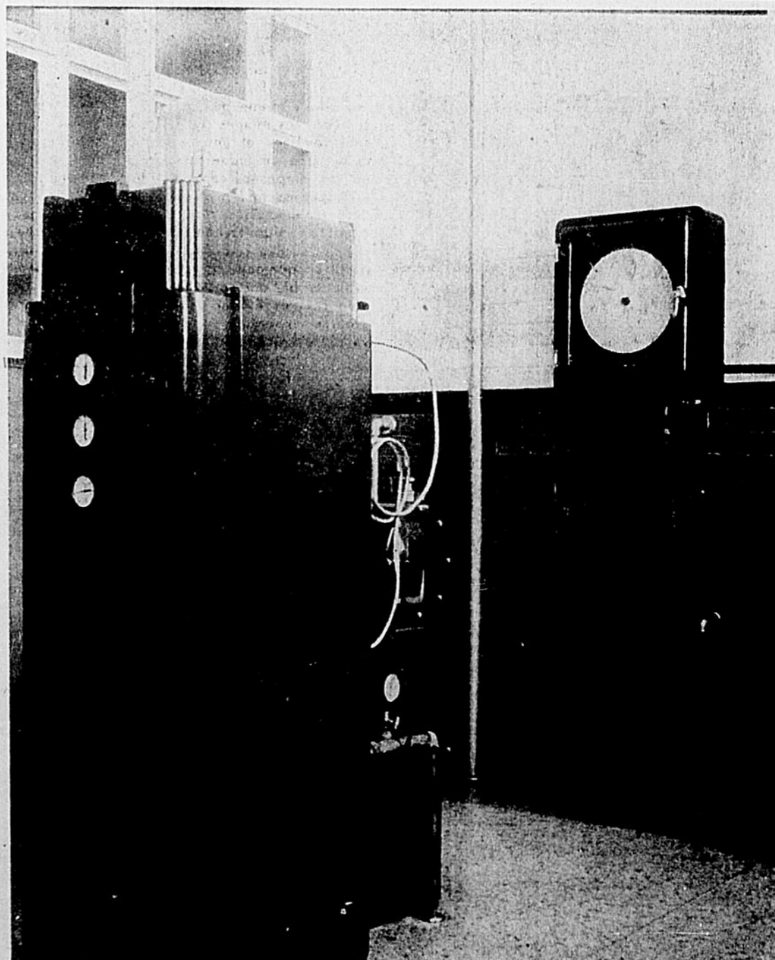
La photo ci-dessus nous offre une vue d'ensemble du nouveau chlorinateur que la ville vient d'acquérir, au coût de $5,900, pour notre usine de
