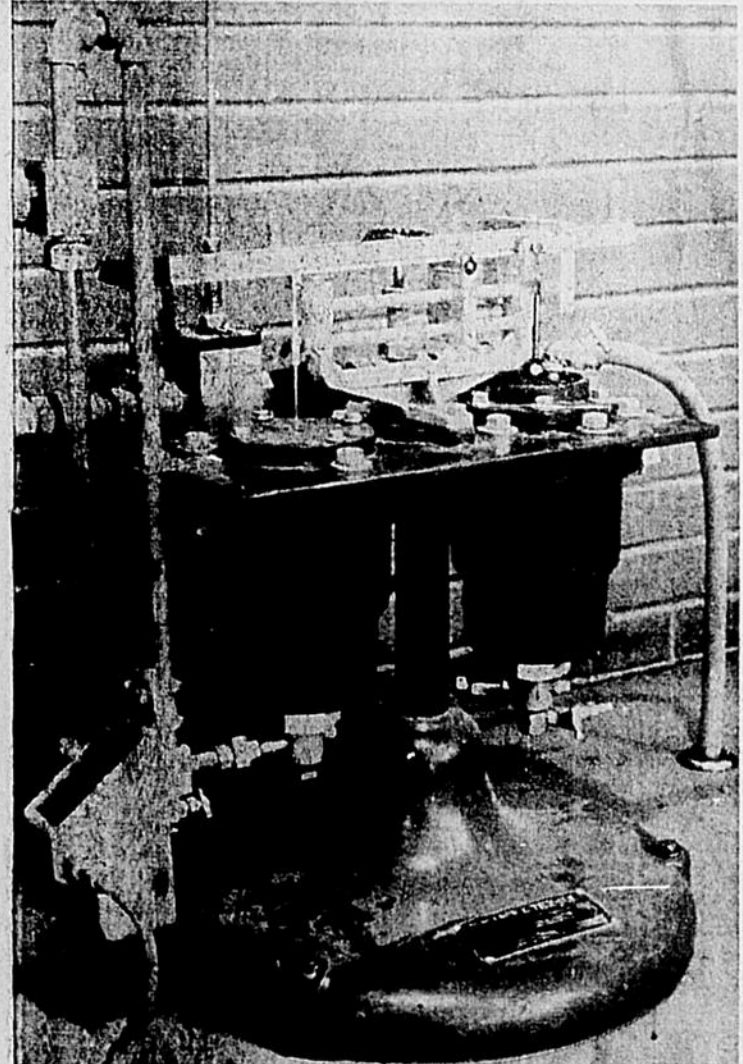
Nous voyons ci-dessus une reproduction photographique de l'appareil de contrôle proportionnel automatique, ajusté sur le tuyau principal venant de la rivière, qui entre dans le procédé de chloration, à l'usine de filtration municipale.
