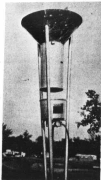
Piège lumineux pour la lutte contre les moustiques, mis au point par l'entomologiste J.-B. Maltais.
