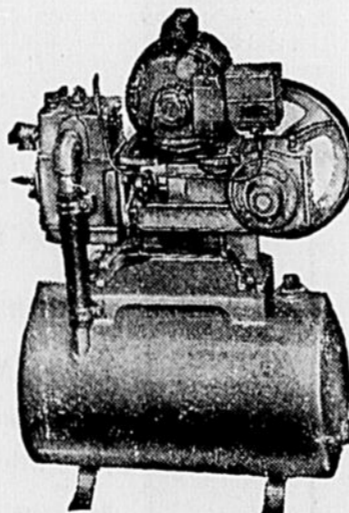
POMPE pour puits de surface, montée sur réservoir horizontal. La pompe a une capacité de 300 gallons à l'heure. Ce modèle est en grande demande. Prix à compter de $142.50
