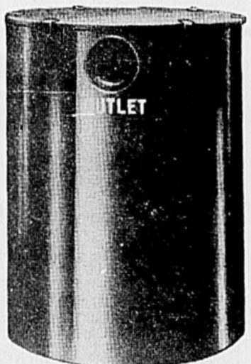
RESERVOIR SEPTIQUE , en acier épais enduit de goudron, pour les endroits où il n'y a pas d'égout sanitaire. Ces réservoirs sont approuvés par le Bureau d'Hygiène. Grandeurs, 36" x 48", 46" x 48", 50" x 60". Prix à compter de $36.00
