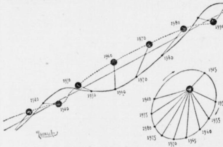
LA FIGURE MONTRE les mouvements des deux étoiles par rapport aux étoiles voisines, et aussi celui du centre de gravité du système. L'éclipse représente le mouvement du Compagnon autour de Sirius (période 50 ans).
