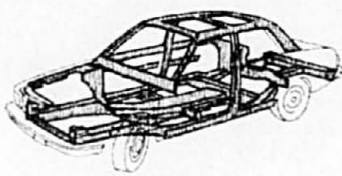
Une cage d'acier aux compartiments déformables protège les passagers.
