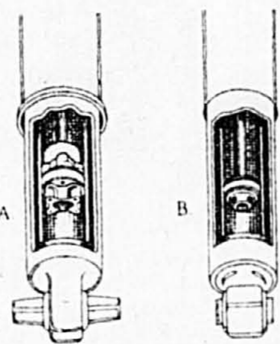
A. Amortisseur arrière de la 505 SR Peugeot et son imposant système de soupapes, qui lui permet de jouer un double rôle - pour le confort, et pour la tenue de route.
