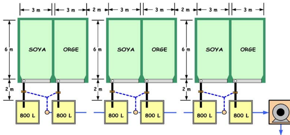
Figure 7.2 : Dispositif expérimental
