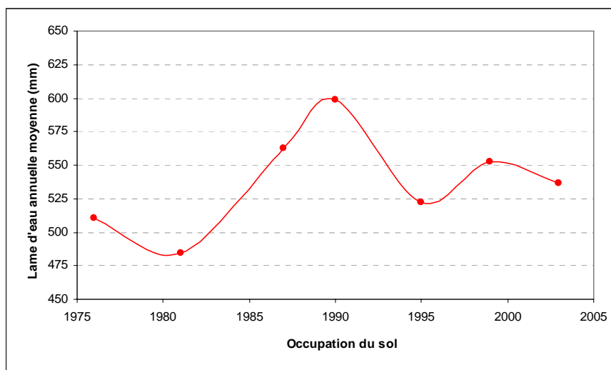
Figure 5.12 : Variation de la lame d'eau annuelle moyenne simulée au niveau du sous-bassin Beurivage en fonction de l'occupation du sol
