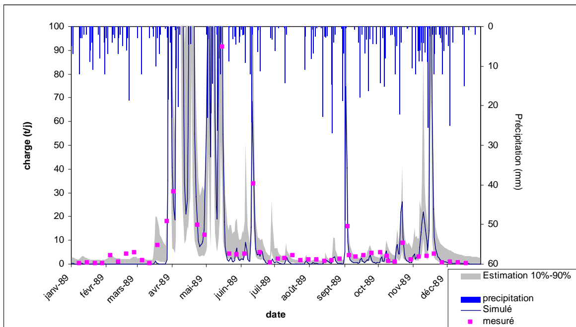
Figure A.2: Comparaison des charges journalières simulées (GIBSI) et observées pour l'année 1989 à l'exutoire de la Beurivage (tronçon 1644)
