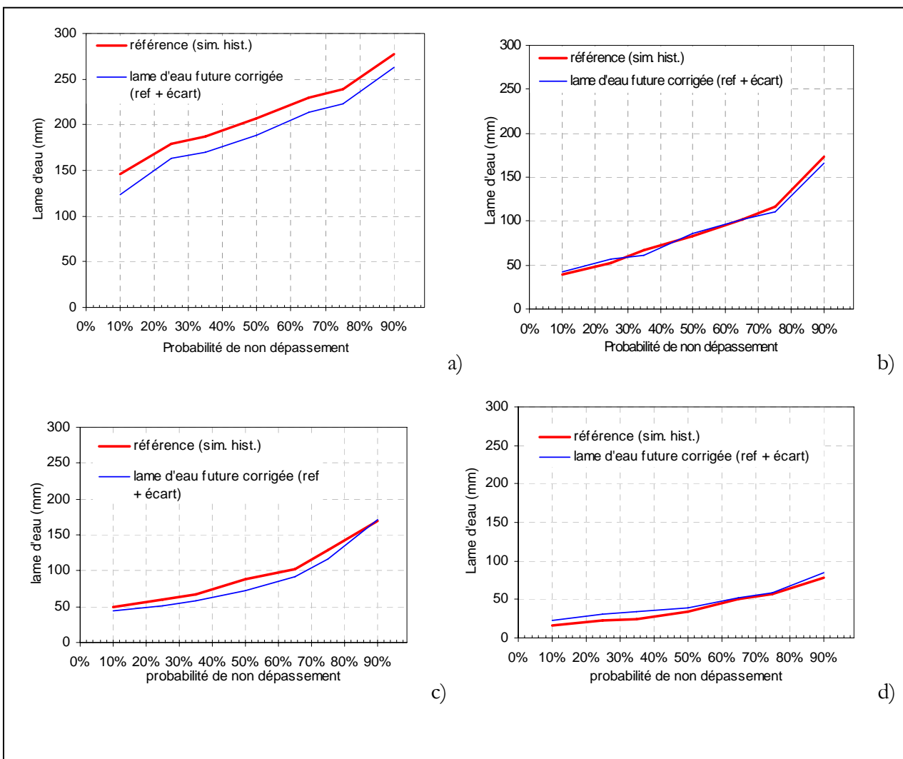
Figure I.8 : Probabilité de non dépassement des lames d'eau simulées à l'exutoire de la Chaudière selon les données historiques et les chroniques des MCG-SEM HadCM3 A2a et B2a « corrigées » appliqués par la méthode du Downscaling, au printemps (a), à l'été (b), à l'automne (c) et à l'hiver (d).
