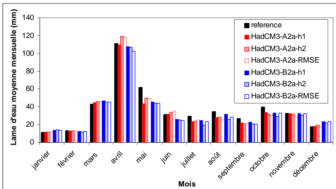
Figure J.2: Lame d'eau mensuelle moyenne (sur les 30 ans) simulée à l'exutoire de la Chaudière avec les données historiques (en noir) et avec les données futures issues des MCG-SEM et chroniques considérés (en rouge)
