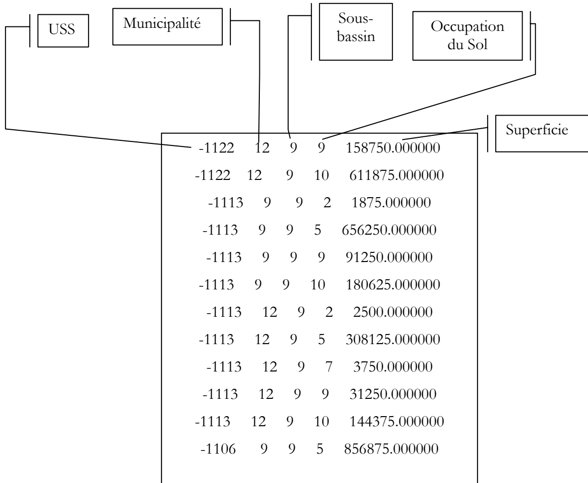
Figure F.4 : Différentes composantes d'un fichier statistique
