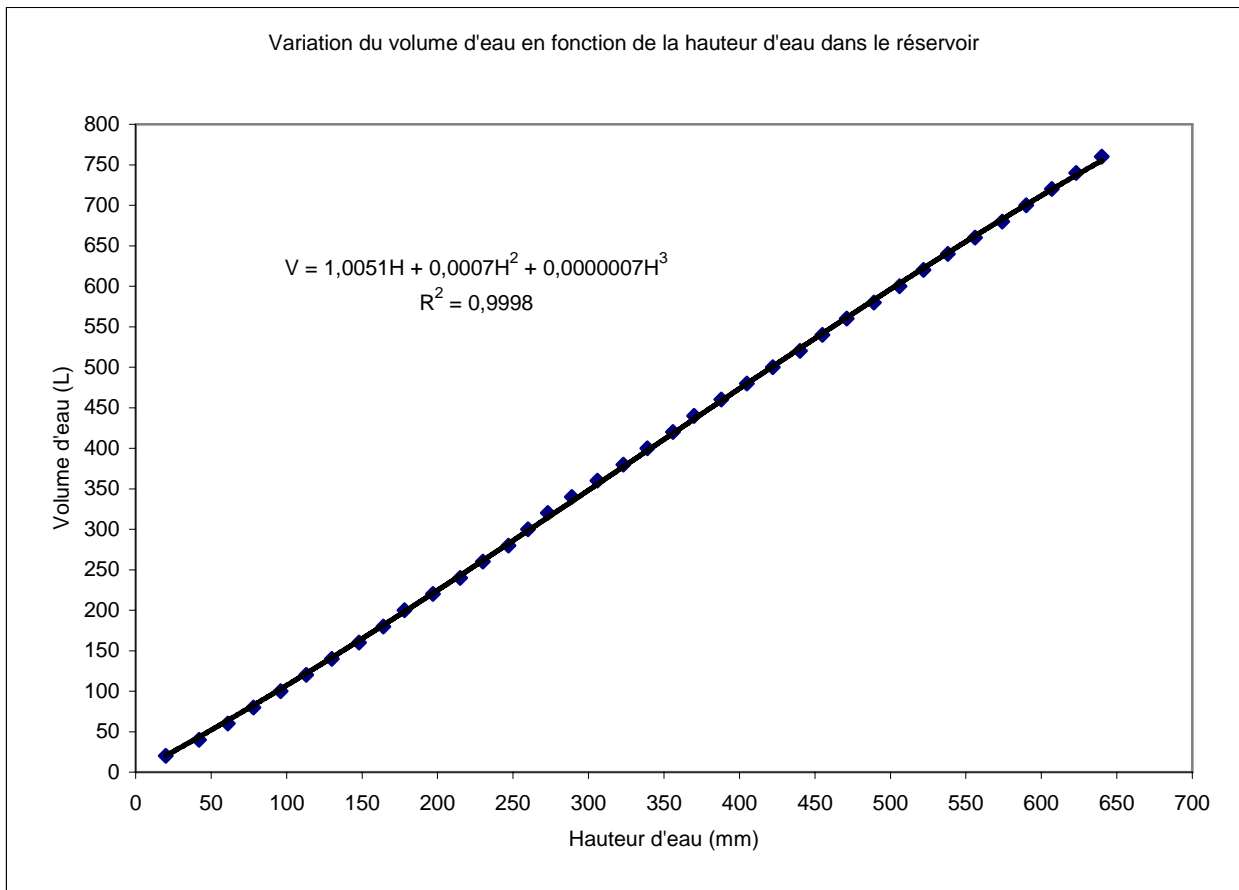
Figure M.1 : Relation entre la hauteur d'eau et le volume d'eau accumulée dans un réservoir.
