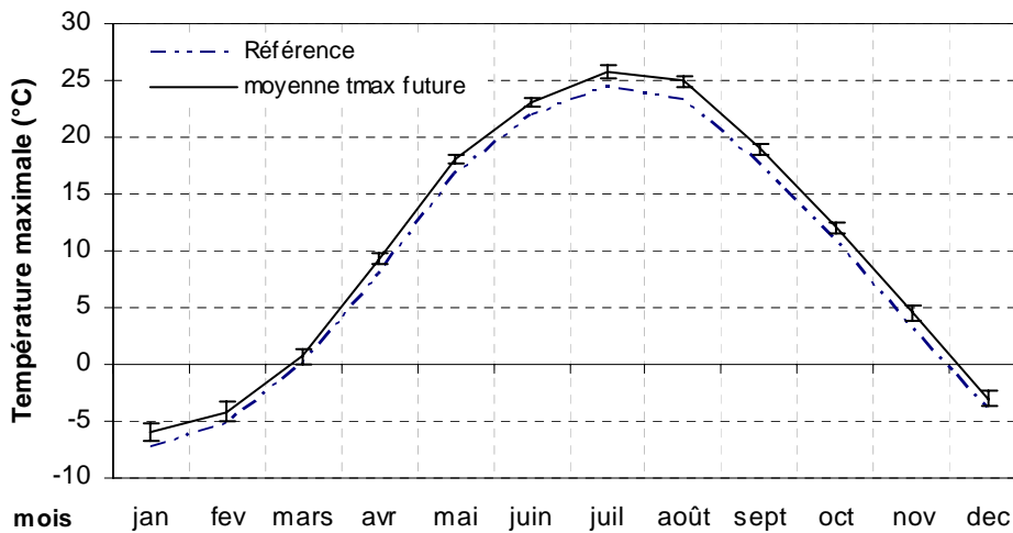
Figure H.9: Évolution de la moyenne mensuelle de la température journalière maximale passée et future tous MCG SEM confondus (moy. ± σ) au cours de l'année à la station de Saint Flavian.
