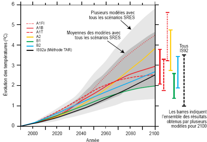
Figure 6.3 : Évolution de la température moyenne mondiale pour les six scénarios indicatifs SRES, dérivée au moyen d'un modèle climatique simple. (Source : Bilan 2001 des changements climatiques : Les éléments scientifiques, Rapport du Groupe de travail I du GIEC, Contribution du Groupe de travail I au troisième rapport d'évaluation du Groupe d'experts intergouvernemental sur l'évolution du climat , page 66)
