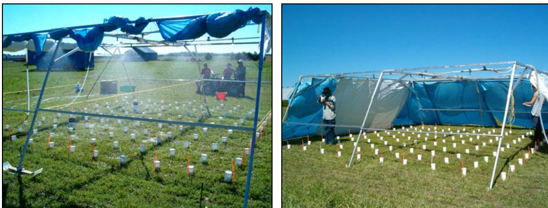
Figure 7.6 : Test d'intensité de pluie et mesure des hauteurs d'eau.
