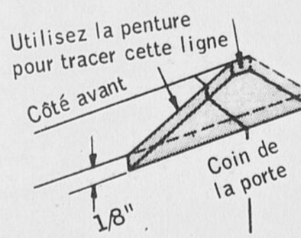
FIG. 5 DETAIL DES MORTAISES REQUISES POUR RECEVOIR LES PENTURES SEMI-INVISIBLES
