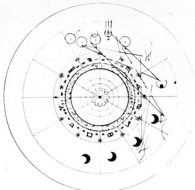
Le ciel de la semaine du 10 au 17 janvier 1979. Telle sera la position de chaque planète.
