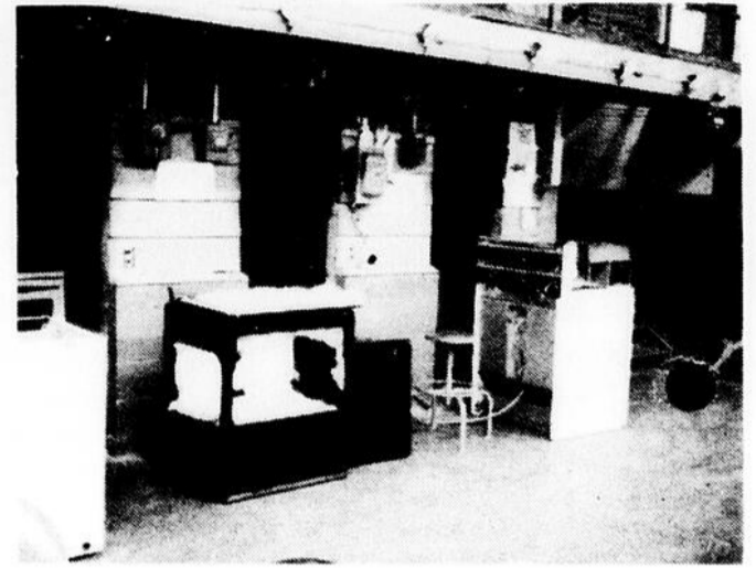
Une sécheuse et une cuisinière électrique en réparation dans le cadre de l'option Electromécanicien en appareils ménagers. [Photo R. Dubé]
