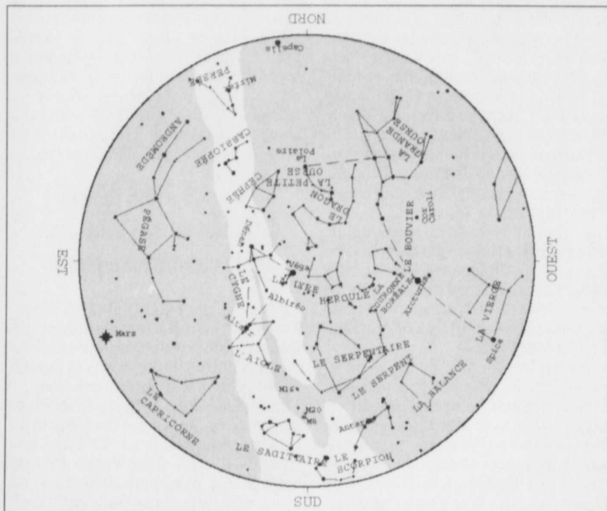
La carte représente le ciel tel qu'on pourra le voir à la mi-juillet vers 23h30, une heure plus tard au début du mois, une heure plus tôt à la fin. Pour utiliser, tenez la carte au-dessus de votre tête, en alignant les points cardinaux. Les lignes pleines identifient les constellations, tandis que la bande claire indique le tracé de la Voie lactée.
