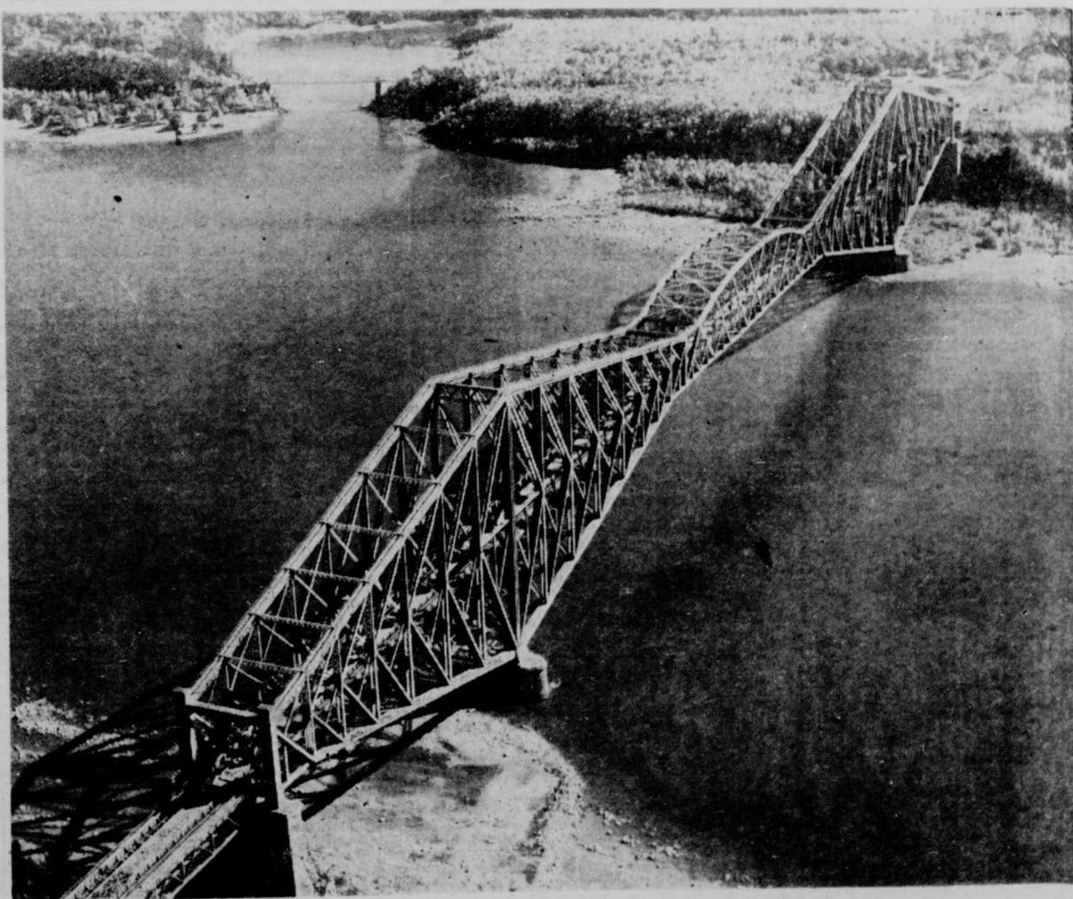
• Vue aérienne du PONT de QUEBEC, considéré, lors de sa construction, comme la huitième merveille du monde. Les premiers plans en vue de la construction d'un pont sur le Saint-Laurent, près de Québec, furent faits en 1852, soit il y a cent ans. Cette oeuvre du génie fut complétée, après deux désastres (1907 et 1916), en 1917. Son inauguration officielle eut lieu le 22 août 1919, par S. A. R. le Prince de Galles, le futur Edouard VIII. — (Voir la note en page 2.)
