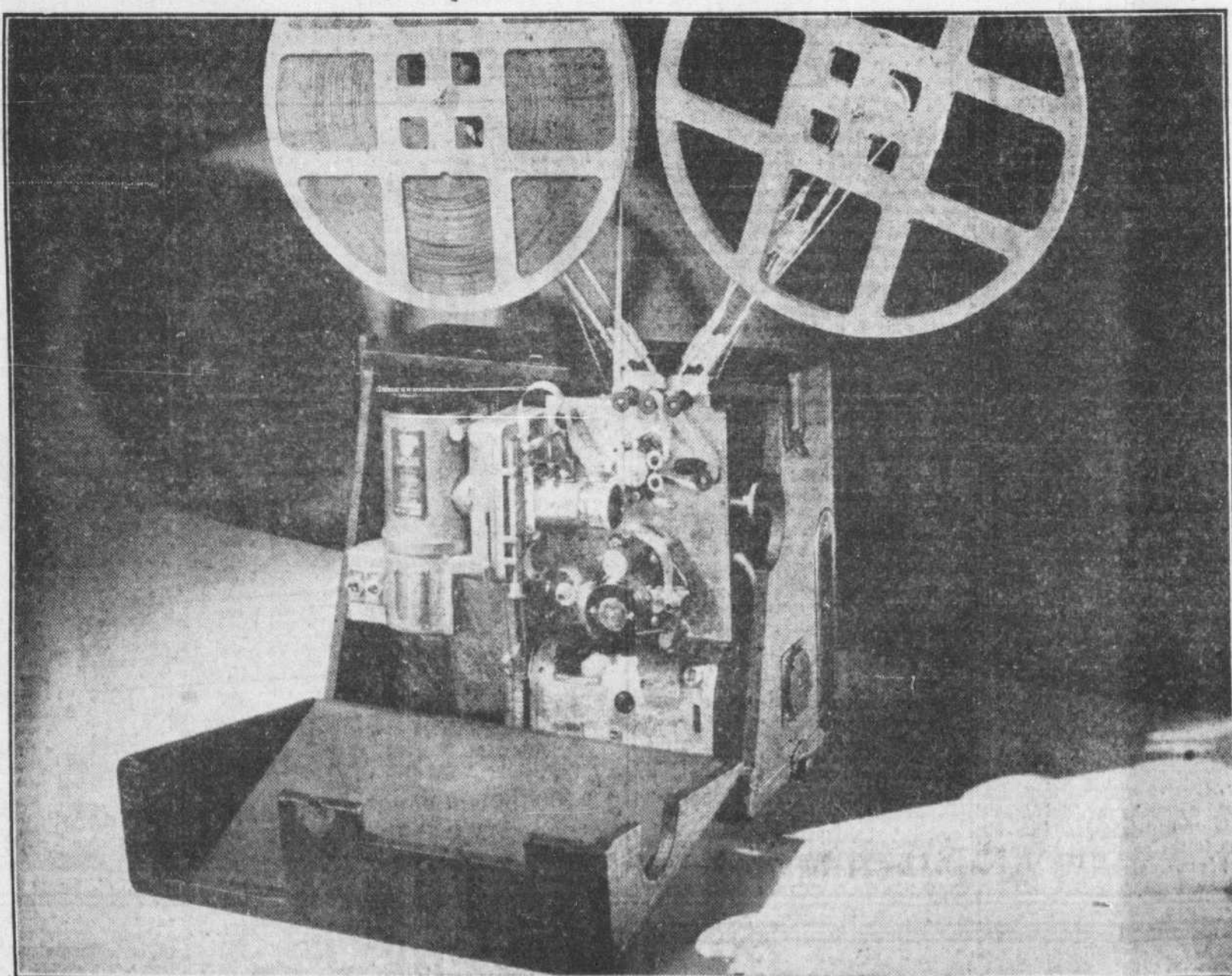
VIGNETTE DU MODELE 40A STANDARD — 1000 WATTS
