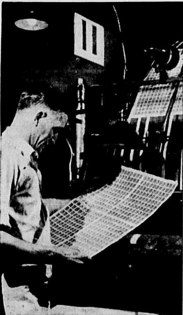
Cette presse imprime environ 1.000 feuilles de timbres en une heure. Le pressier vérifie la distribution de l'encre et l'œil électrique que l'on peut apercevoir sur la photo compte sans jamais se tromper le nombre de feuilles qui sortent de la presse.
