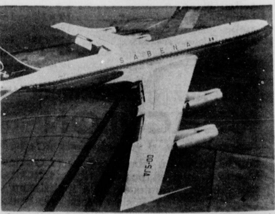
Cette vue plongeante du Boeing 707 permet de voir les volets baissés à 45 degrés. De chaque côté se trouvent les gouvernails de profondeur qui permettent de guider l'avion dans le ciel et à terre. L'avion vient de se poser. On peut voir le gouvernail de profondeur de droite baissé et celui de gauche relevé. L'avion a amorcé un virage au sol pour rejoindre l'aire de débarquement. Les obstrucateurs d'air se trouvent sur l'aile avant, entre les moteurs.
