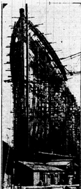
Une magnifique scène du nouveau géant de la mer, le No. 534, que l'on est en train de terminer aux chantiers navals de Clydebank, à Glasgow.
