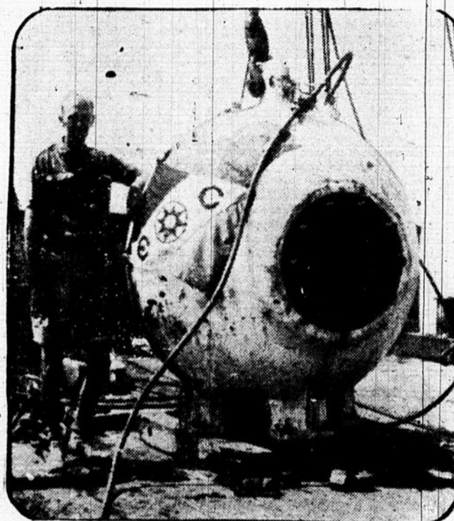
Dr. WILLIAM BEEBE, explorateur américain, que l'on voit dans la photo près du ballon d'acier dans lequel il a descendu à 2,510 pieds sous la mer. Il était accompagné de Otis Barton lors de sa descente d'un demi-mille sous la mer, et il assure avoir trouvé un poisson qui ressemblait à un arbre de Noël. L'explorateur américain a établi un record, l'ancienne marque étant de 2,200 pieds.
