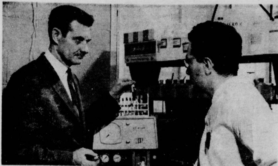
Le docteur Jean - Paul DuRuisseau D.Sc., et monsieur Gabriel El Kouri, M.Sc., devant un appareil d'absorption atomique servant à mesurer le magnésium.
