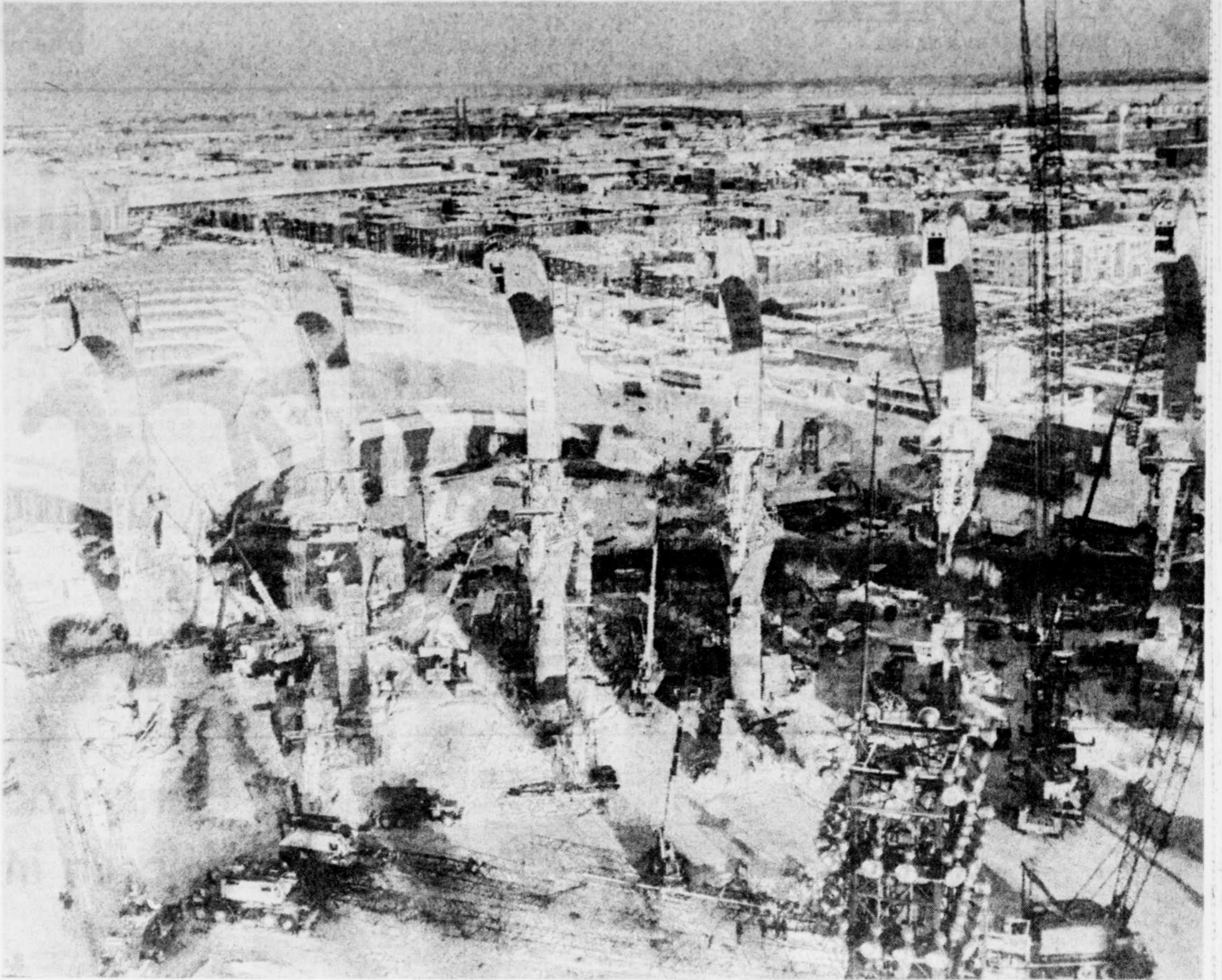
Les 38 poutres sont érigées mais l'anneau reste encore à construire.
