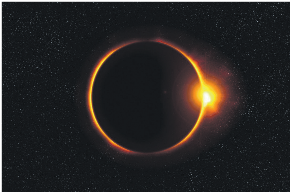
Éclipse solaire. Photo Pixabay
