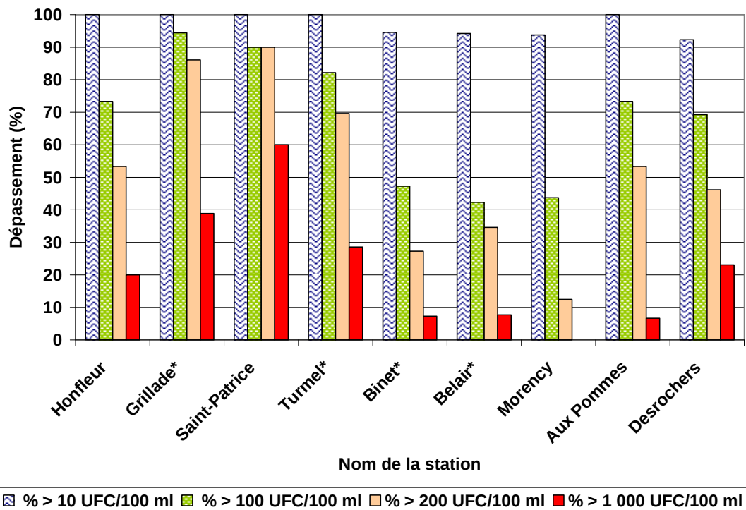
Figure 4 Dépassement des seuils de CF en été aux stations des régions hydrographiques 02 – Saint-Laurent sud-est et 05 – Saint-Laurent nord-ouest pour la période de 2003 à 2005 (de 1999 à 2001 aux quatre stations suivies d'un astérisque)
