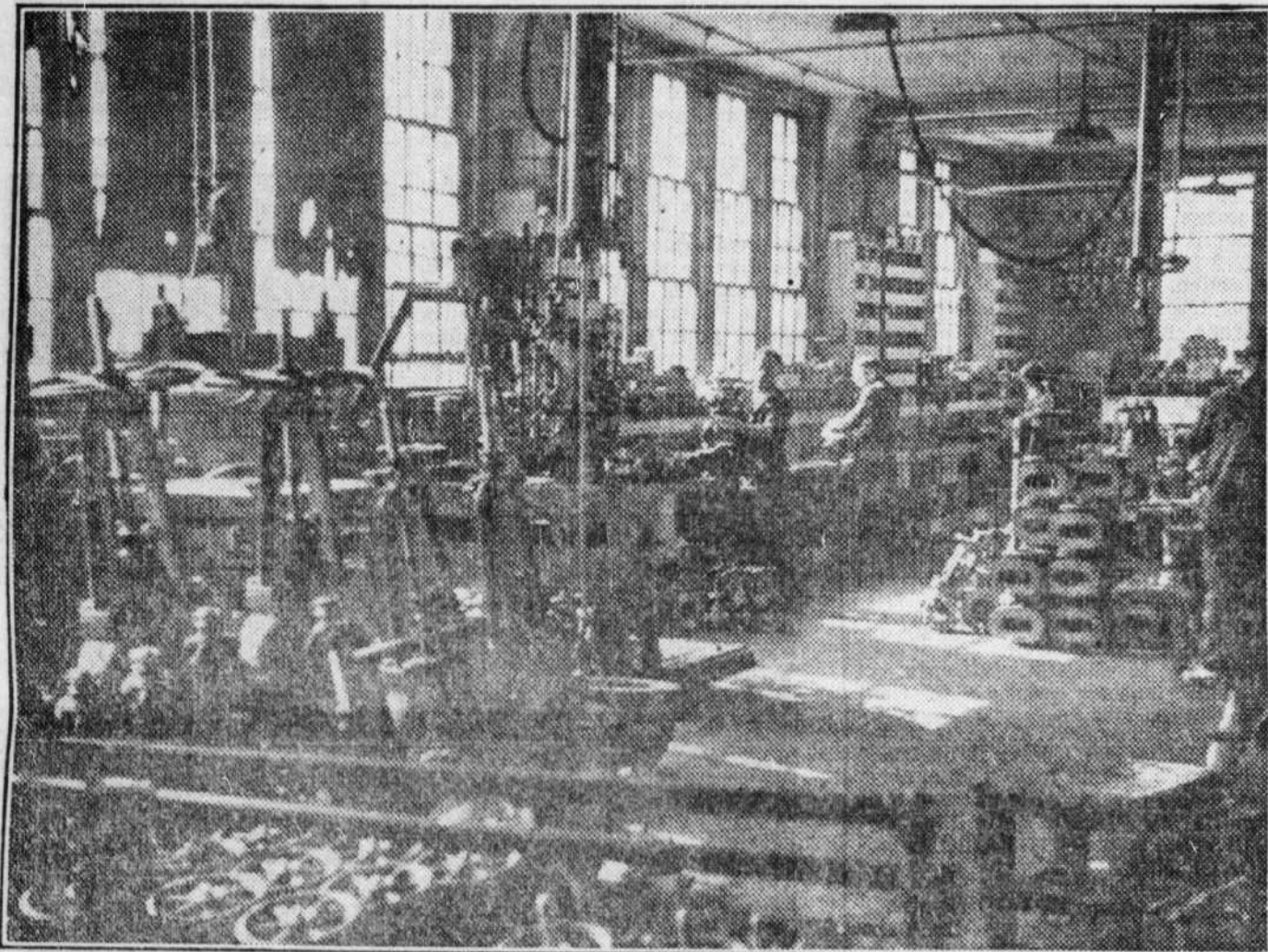
Où les robinets Crane sont essayés et examinés.
