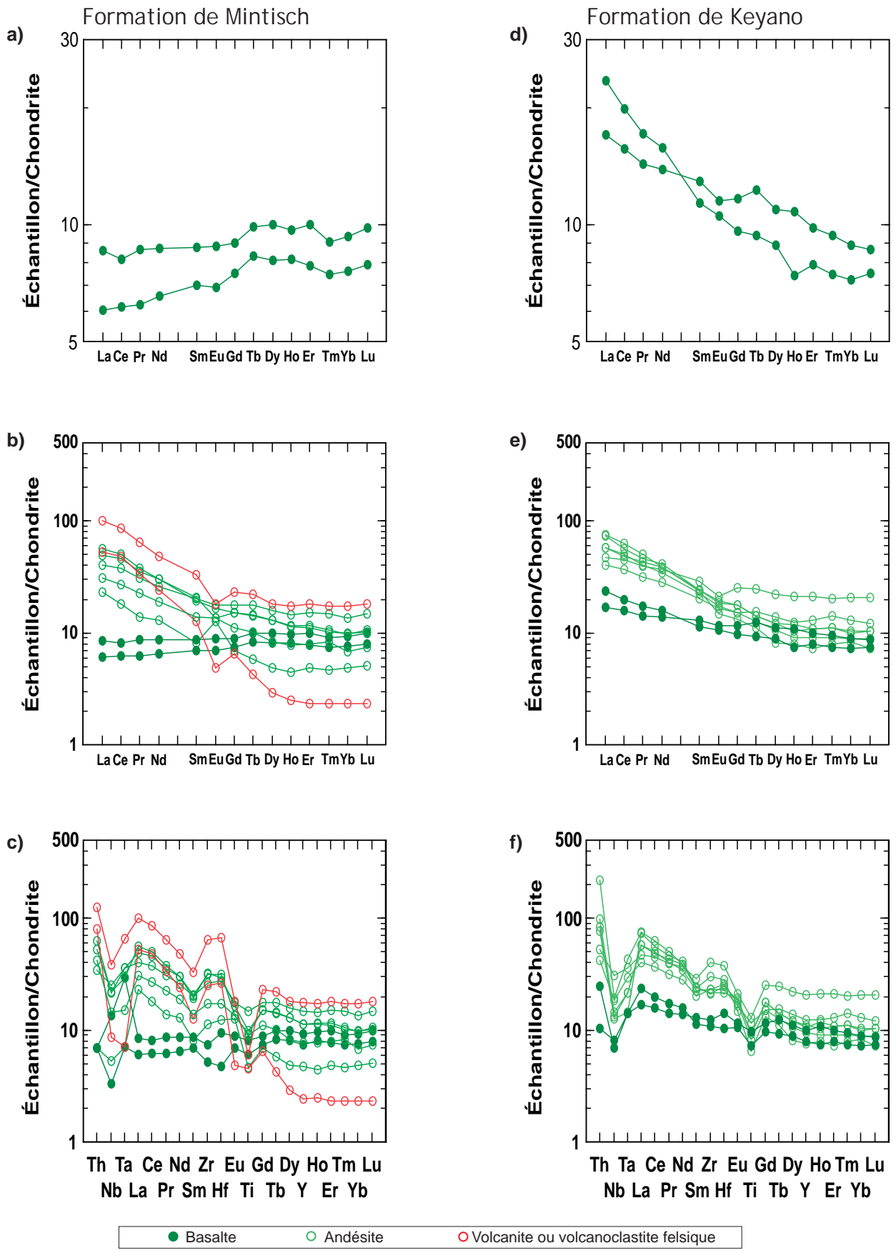
FIGURE 7 – Diagrammes des éléments des terres rares et multiéléments normalisés aux valeurs des chondrites C1 de Sun et McDonough (1989) : a), b) et c) Formation de Mintisch; d), e) et f) Formation de Keyano
