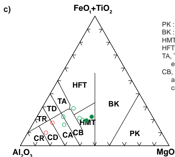
FIGURE 5 – Diagrammes de caractérisation géochimique de roches volcaniques des formations Mintisch et Keyano : a) et d) diagrammes de classification \text{SiO}_2 vs \text{Zr/TiO}_2 \times 0,0001 (Winchester et Floyd, 1977); b) et e) diagrammes d'affinité magmatique (Ross et Bédard, 2009); c) et f) diagrammes ternaires cationiques ( \text{FeOt} + \text{TiO}_2 ) - \text{Al}_2\text{O}_3 - \text{MgO} (Jensen, 1976).
