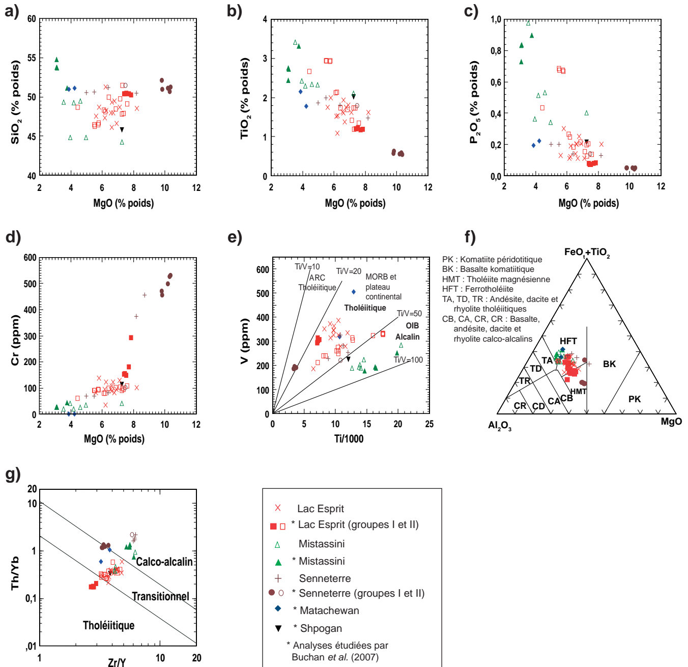
FIGURE 14 – Diagrammes de caractérisation géochimique des dykes mafiques néoarchéens et paléoprotozoïques: a) , b) , c) et d) des éléments majeurs SiO 2 , TiO 2 , P 2 O 5 et Cr en fonction de MgO; e) de Shervais (1982); f) de Jensen (1976); g) de Ross et Bédard (2009).
