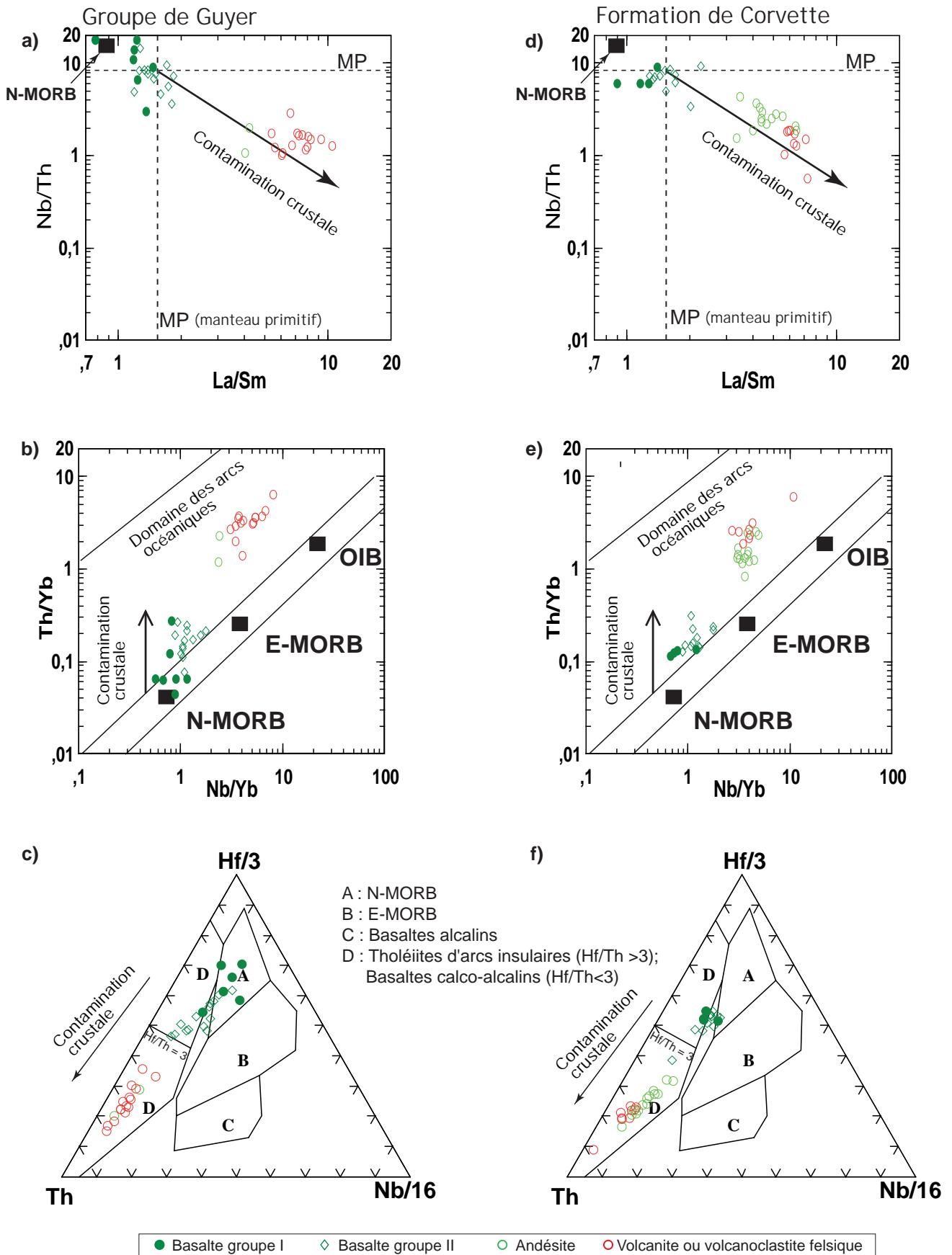
FIGURE 8 – Diagrammes de discrimination et d’environnements géotectoniques pour les roches volcaniques du Groupe de Guyer et de la Formation de Corvette : a) et d) Nb/Th versus La/Sm; b) et e) Th/Yb vs Nb/Yb (Pearce, 2007); c) et f) Th-Hf/3-Nb/16 (Wood, 1980).
