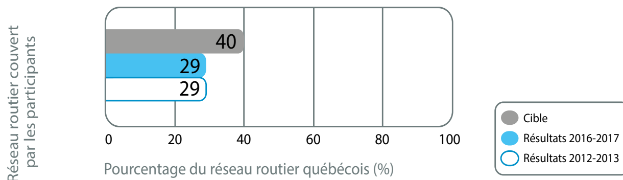
Figure 2 – Pourcentage du réseau routier québécois couvert par les administrations participantes
