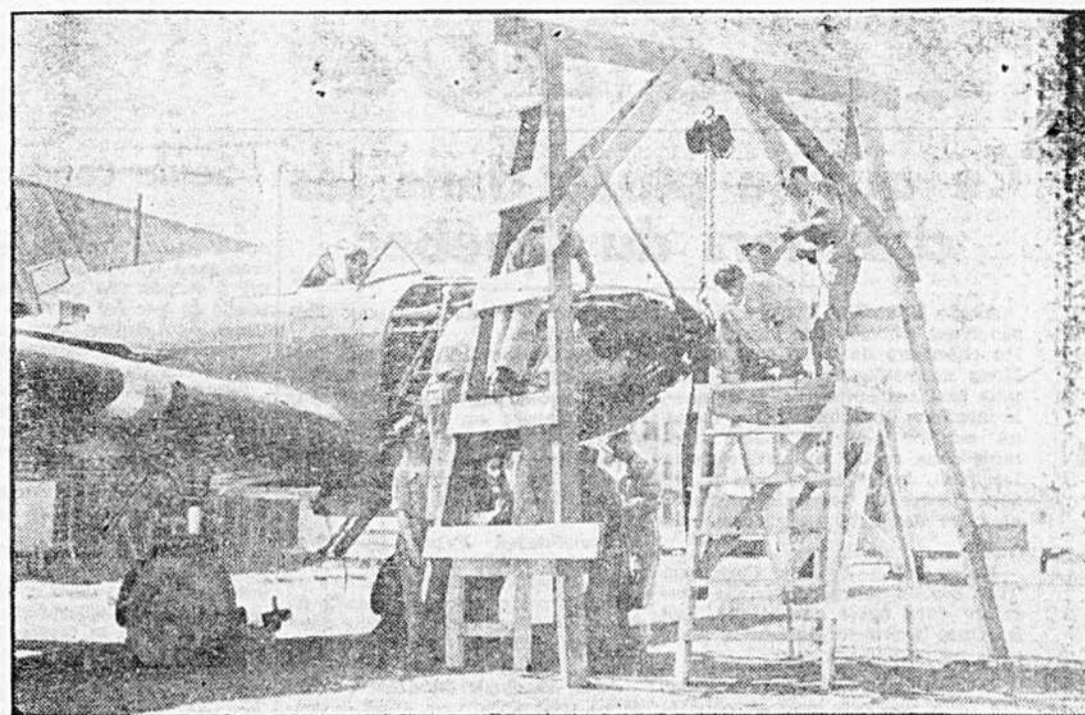
À l'école No 1 d'entraînement technique, de St-Thomas, Ont., des mécaniciens sont en train d'enlever d'un avion de combat "Fairley Battle", un moteur britannique "Merlin" Rolls-Royce. Dans cette institution, on enseigne aux recrues comment fonctionnent les moteurs d'avions et comment on peut les défaire et les monter, pièce par pièce.
