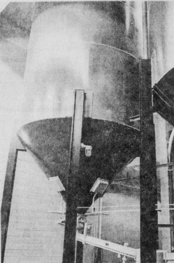
SILLO A CHAUX — La photo nous montre l'un des deux immenses silos à chaux d'une capacité de 3,500 pieds cubes chacun. La chaux sert à enlever l'agressivité de l'eau pour ainsi la rendre neutre.
