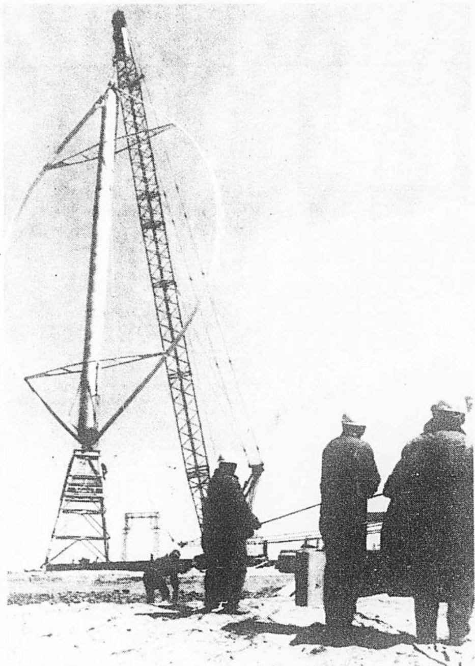
Voici l'allure qu'avait la génératrice éolienne avant que le vent ne la renverse. Elle avait été installée en 1977, par l'Hydro-Québec.
