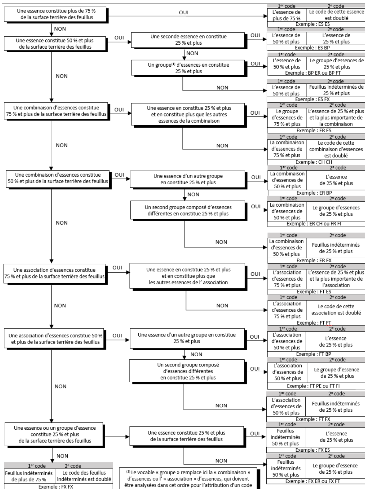
Figure 13. Logigramme 7, peuplement feuillu de 4 m et plus
