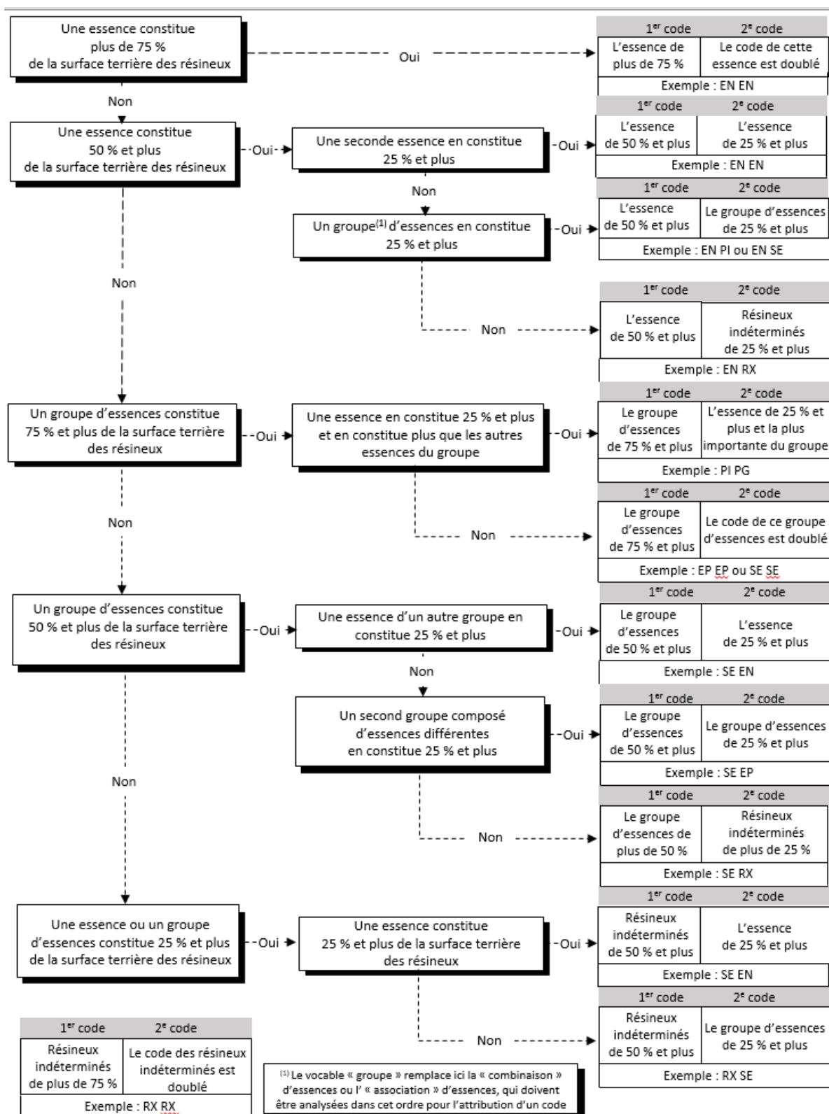
Figure 11. Logigramme 4, peuplement résineux de 4 m et plus
