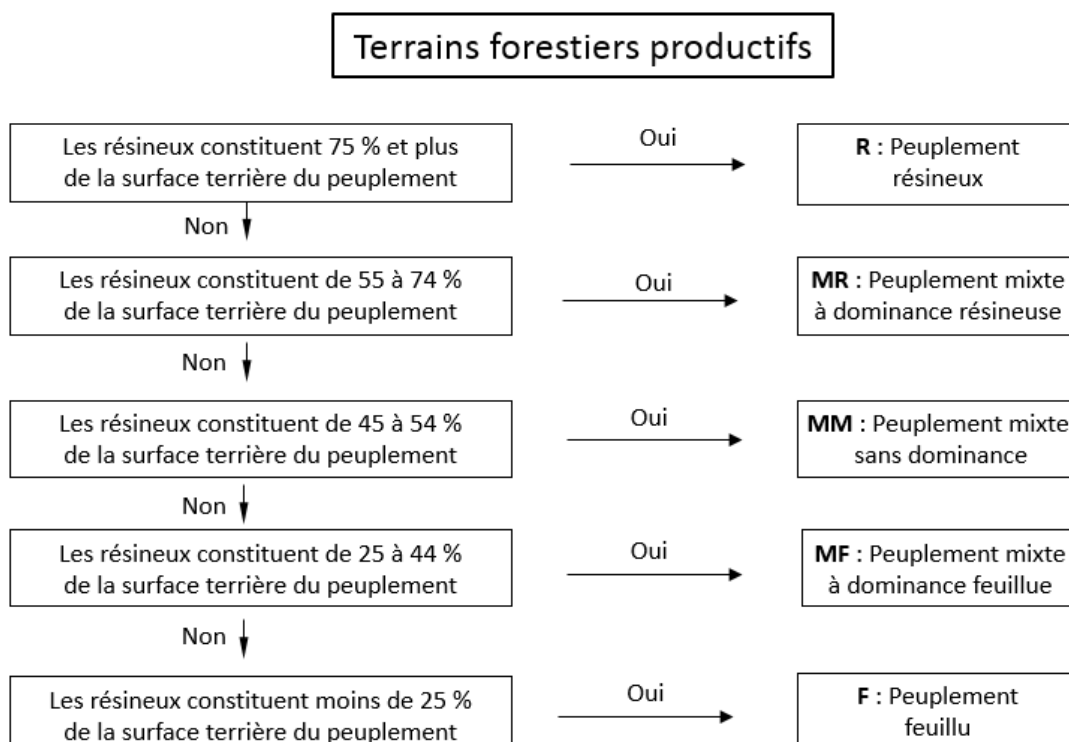
Figure 5. Détermination du type de couvert forestier
