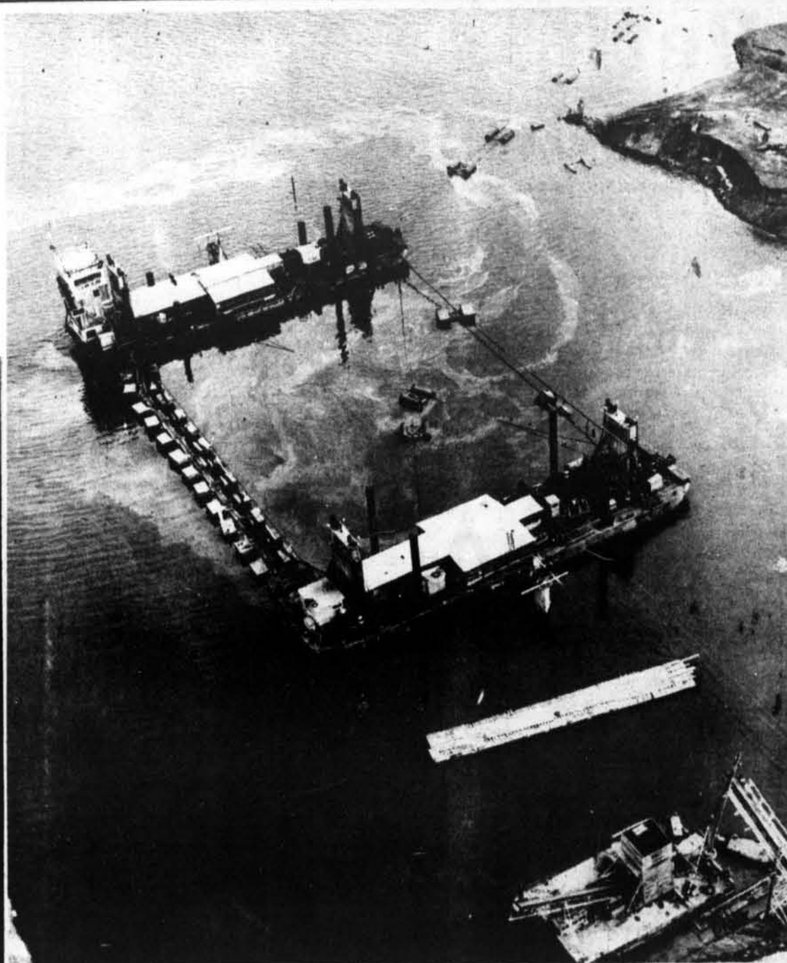
L'ECHOUEMENT, EN PLEINE ACTION, DU SEPTIEME ET DERNIER ELEMENT DU PONT-TUNNEL LOUIS-HILLOLYTE LAFONTAINE PRES DE LA RIVE-NORD DU ST-LAURENT.
