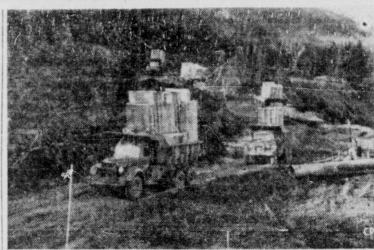
ROUTES DE PORTAGE — Les routes de portage qui longent le tracé de chemin de fer de 360 milles vers le cœur de l'Ungava sont achalandées de camions qui transportent le matériel nécessaire à l'exécution de la grande entreprise. On voit ci-haut des camions, partis de grand matin du camp du millage 28, qui transportent des sections de bâtiments fabriqués d'avance vers un nouvel emplacement de camp. Des tracteurs se tiennent à l'alerte ici et là le long du parcours afin d'aider les camions à se tirer de vilains trous de boue.
