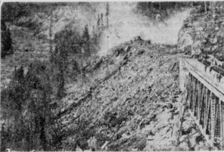
PONT DE LA MOISIE — La rivière Moisie, autre grand obstacle dans l'exploitation des gisements de minerai de fer Labrador-Ungava, est enfin franchie. Un pont d'acier de 708 pieds, sur lequel, un jour, des wagons chargés de minerai pourront circuler, s'étend de l'extrémité d'un tunnel de 2,200 pieds que l'on a pratiqué au travers le roc solide. Ici la rivière Moisie tourne à angle droit.
