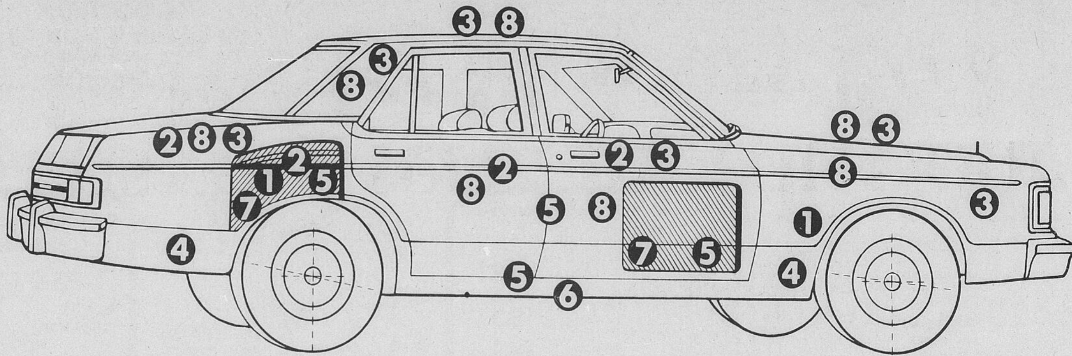
La section en coupe ombrée à l'arrière montre les procédés anti-rouille utilisés à l'intérieur du panneau latéral, près des passages de roue.
