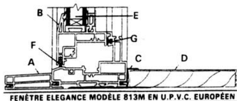
FENÊTRE ELEGANCE MODÈLE 813M EN U.P.V.C. EUROPÉEN
