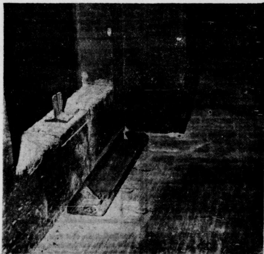
BONNE MANIERE: Les bouts de channels, quand ils sont enlevés de la cuve, doivent être placés par terre et le long du mur, quand c'est du côté extérieur de la bâtisse. Quand c'est au milieu de la bâtisse, ils doivent être placés à plat par terre et au centre de la ligne, c'est-à-dire, vis-à-vis les colonnes.
