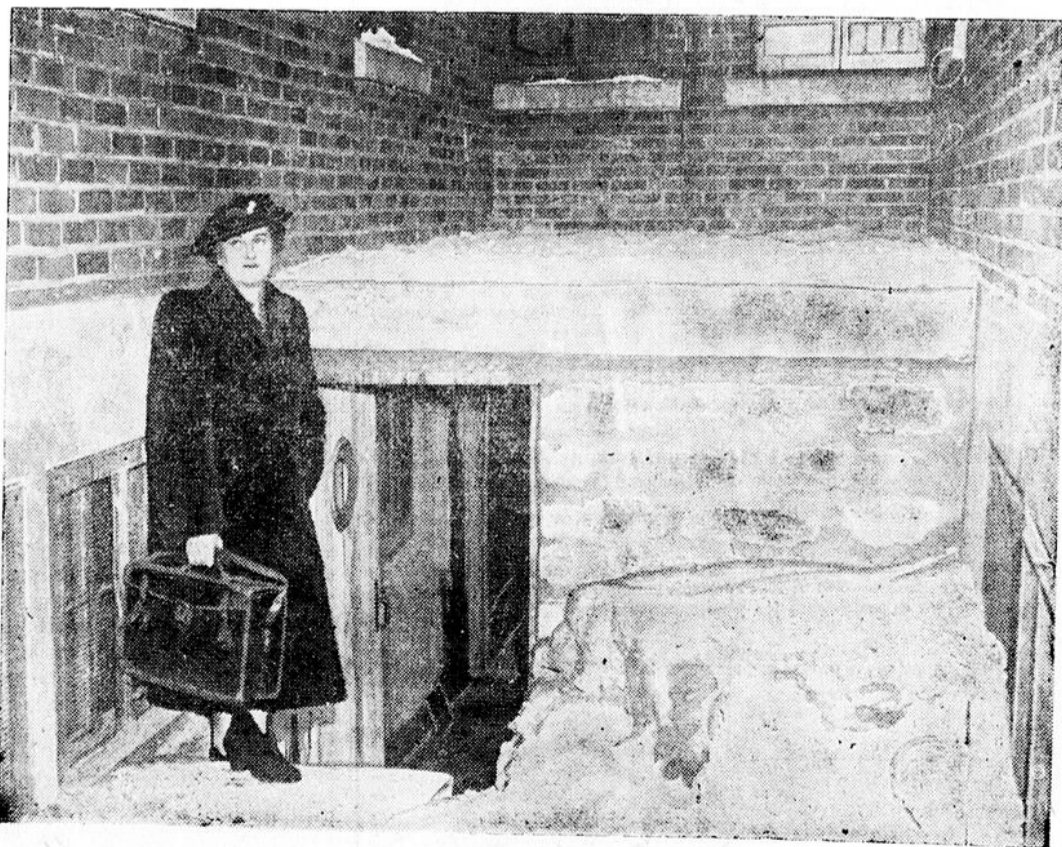
● Il en coûte de $100 à $150 à Montréal pour construire un abri contre les raids. Cette photo nous en montre un qui a été construit récemment. On dit que plusieurs montréalais ont l'intention de s'en faire construire dans le même genre.
