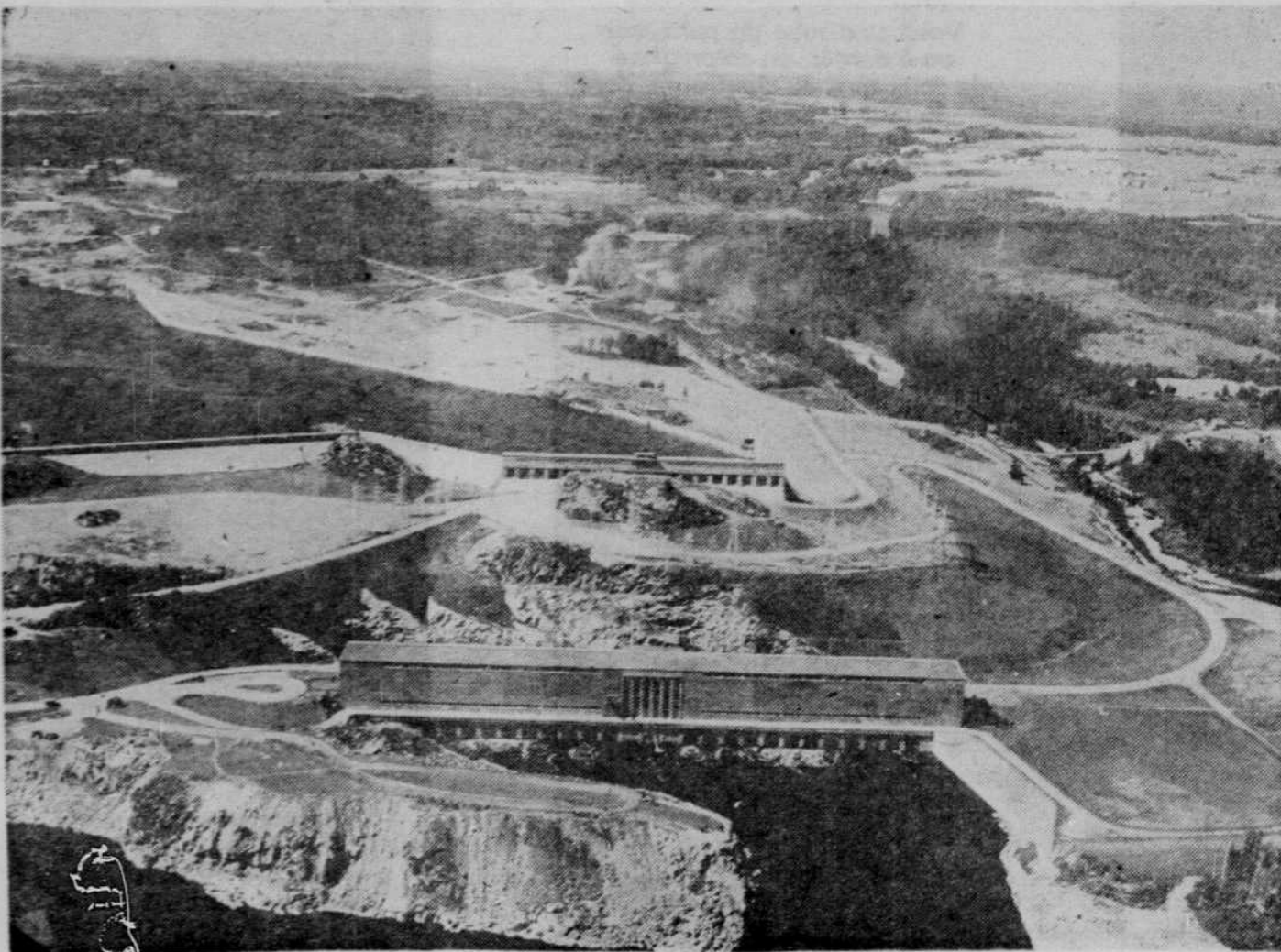
L'aménagement hydro-électrique de Shipshaw.
