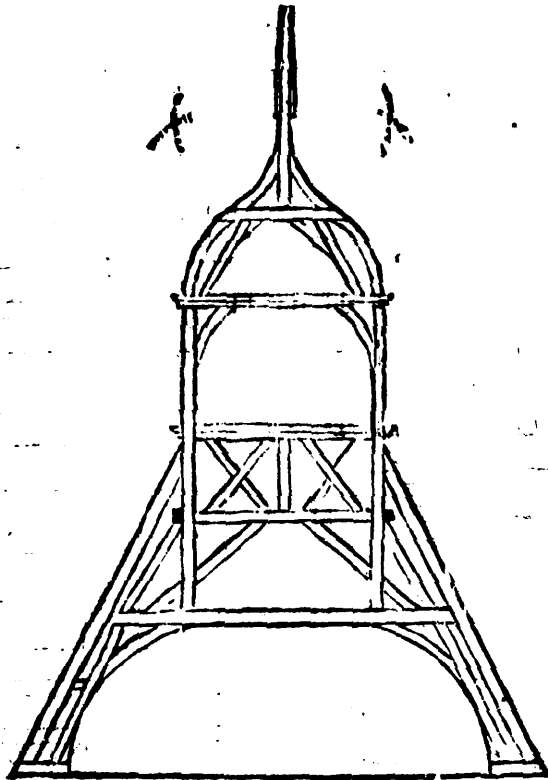
EXPLICATION DE LA LXXV. ET LXXVI. FIGURE Qui montrent la Charpente d'un Dome ou Imperiale.
