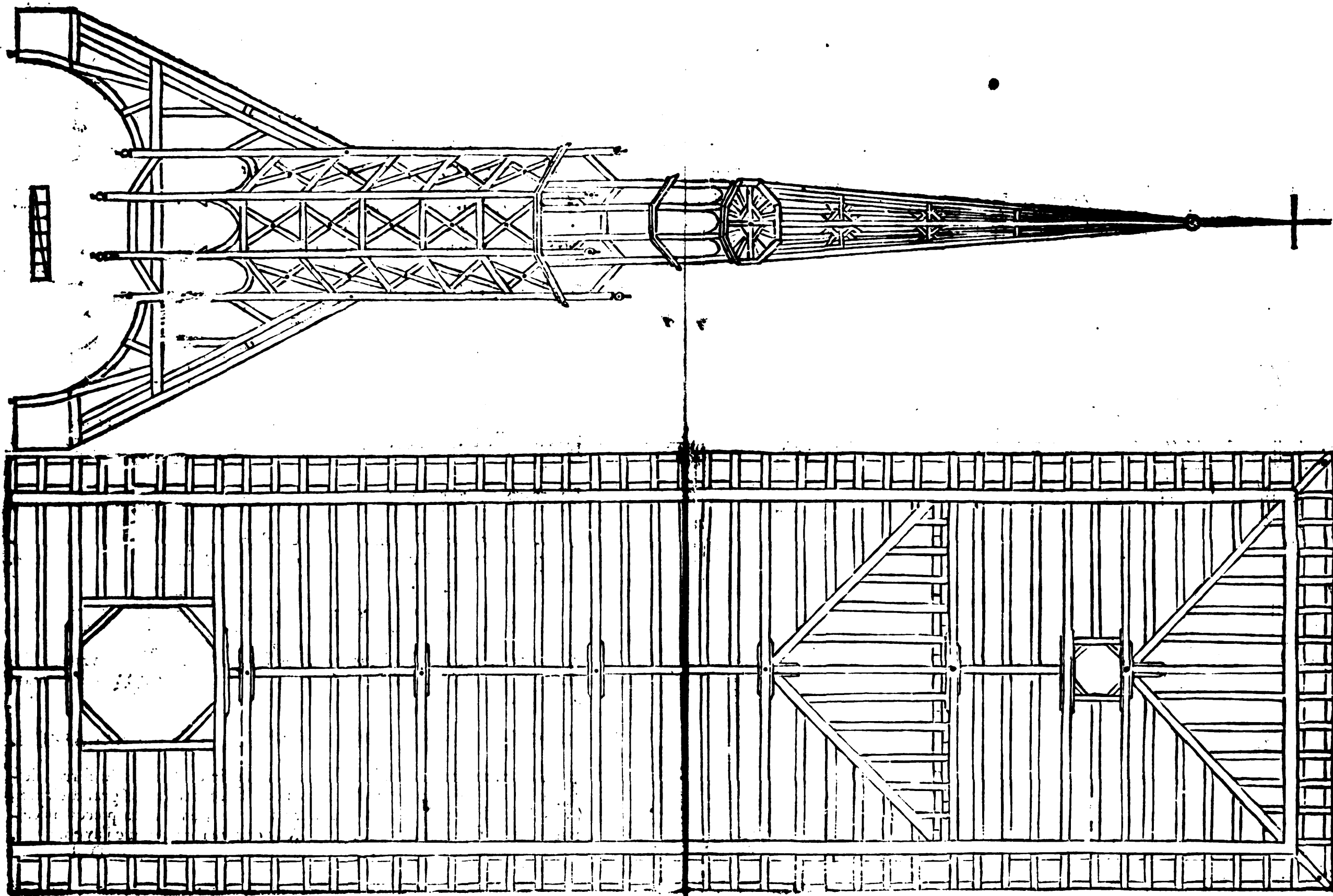
CIV ET CV. FIGURE.
