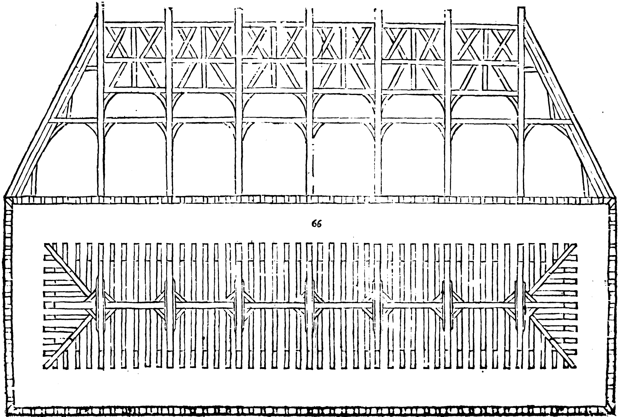
LXVI ET LXVII. FIGURE.
