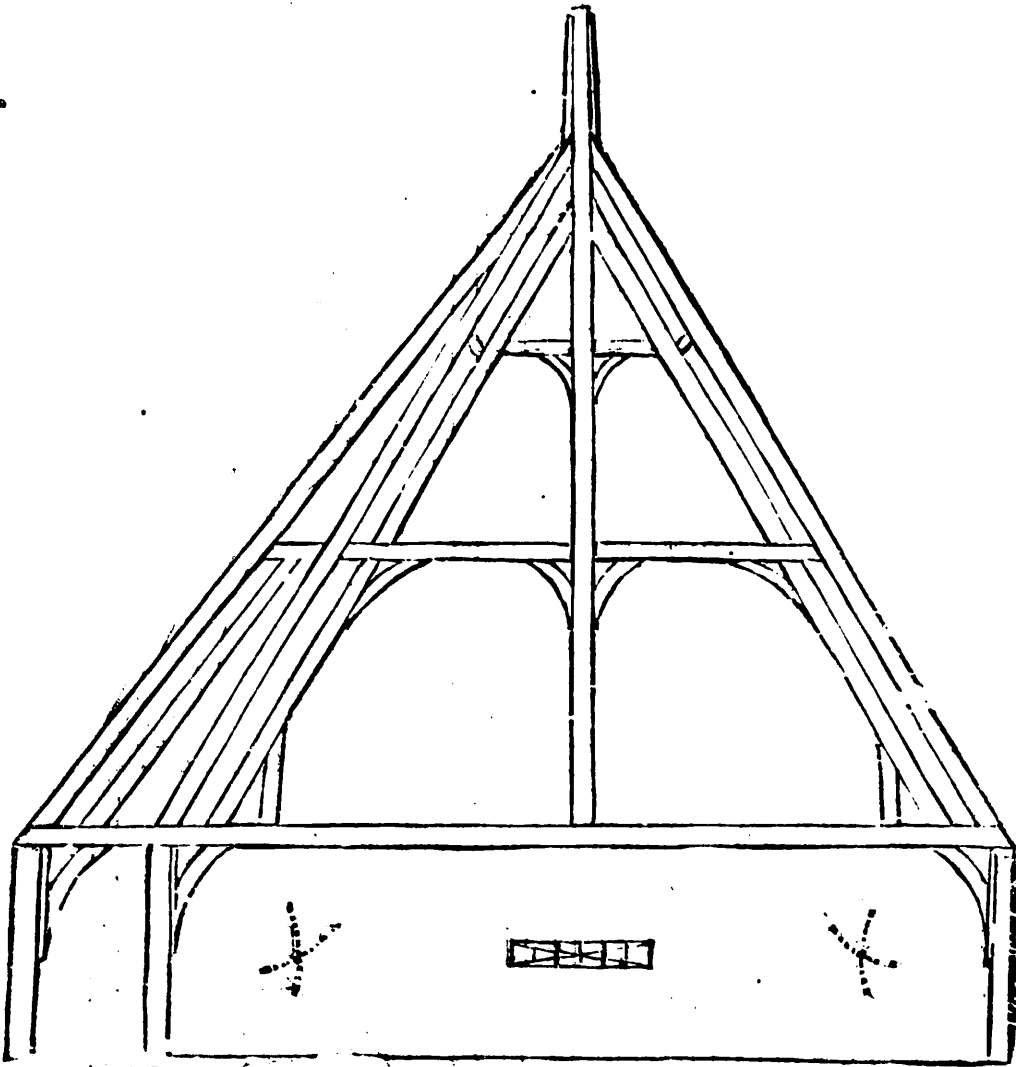
EXPLICATION DE LA LXIX. LXX. LXXI ET LXXII. FIGURES Qui montrent la Charpente d'un Palais, ou Hale.
