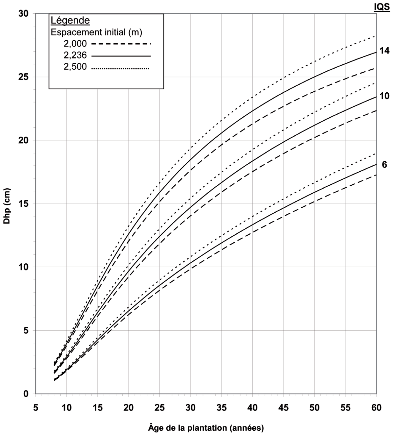
Figure 8. Dhp quadratique moyen estimé à partir des modèles des tables de rendement selon divers IQS et espacements initiaux, pour les plantations d'épinette blanche.
