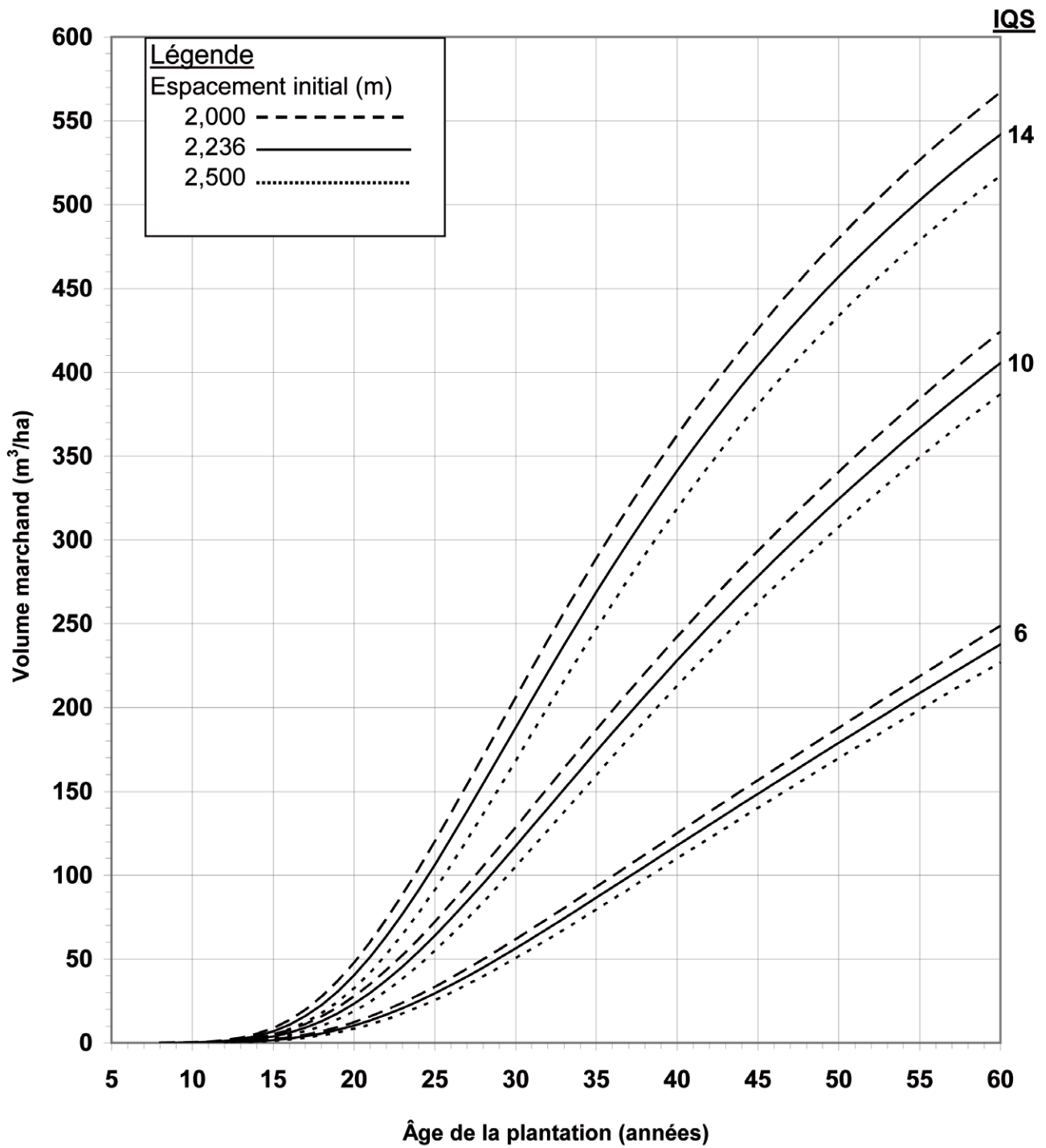
Figure 7. Volume marchand estimé à partir des modèles des tables de rendement selon divers IQS et espacements initiaux, pour les plantations d'épinette blanche.
