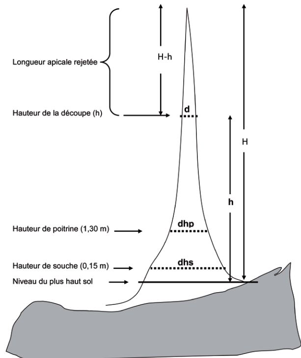
Figure 1. Schéma d'une tige, codification et signification des variables associées au tarif de cubage.
