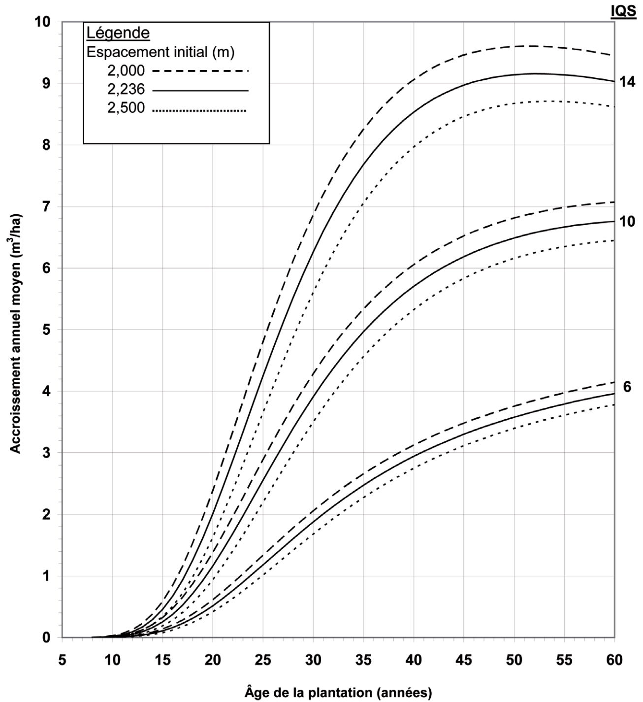
Figure 10. Accroissement annuel moyen en volume marchand estimé à partir des modèles des tables de rendement selon divers IQS et espacements initiaux, pour les plantations d'épinette blanche.
