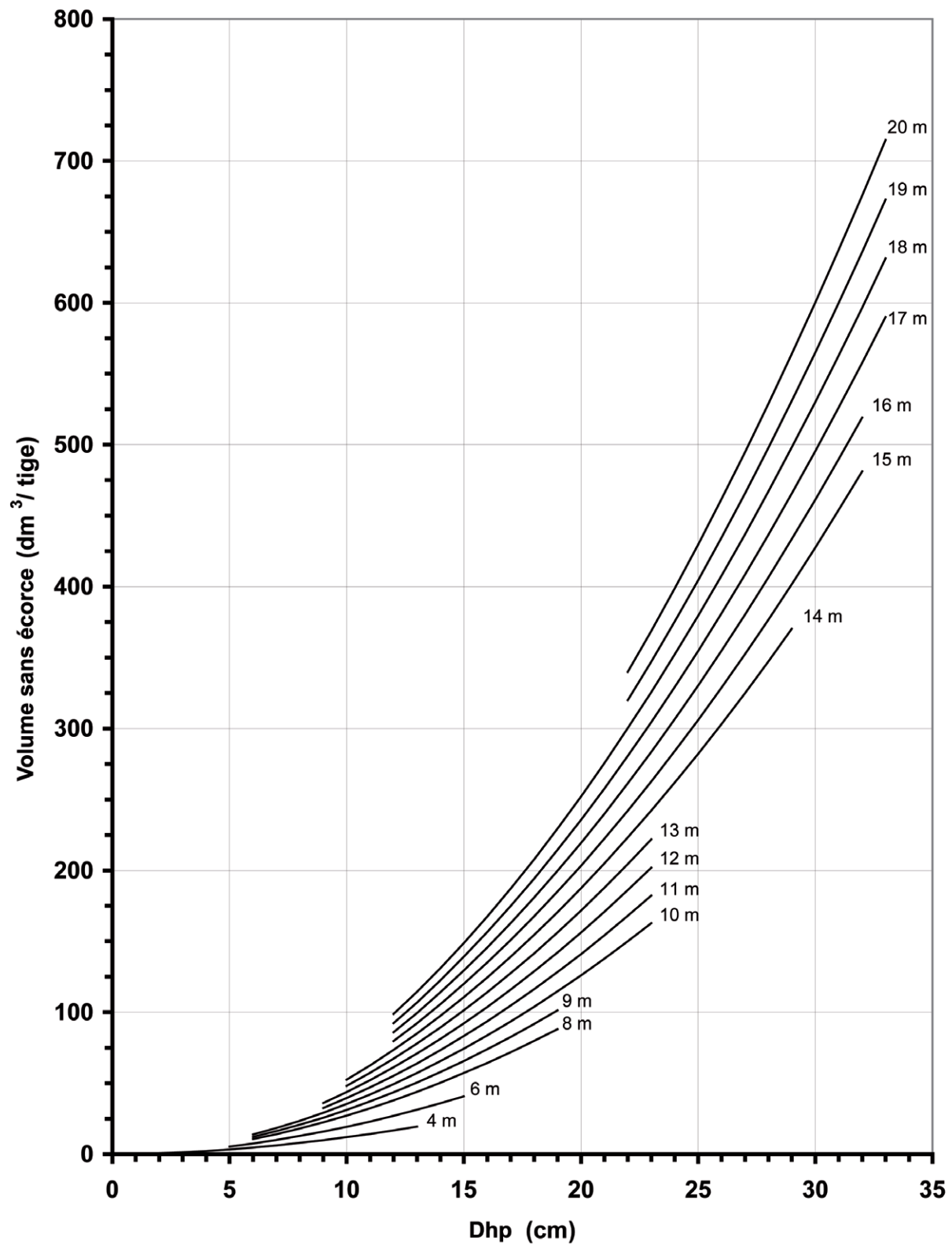
Figure 2. Volume total sans écorce d'une tige d'épinette blanche en plantation en fonction du dhp et de la hauteur totale.
