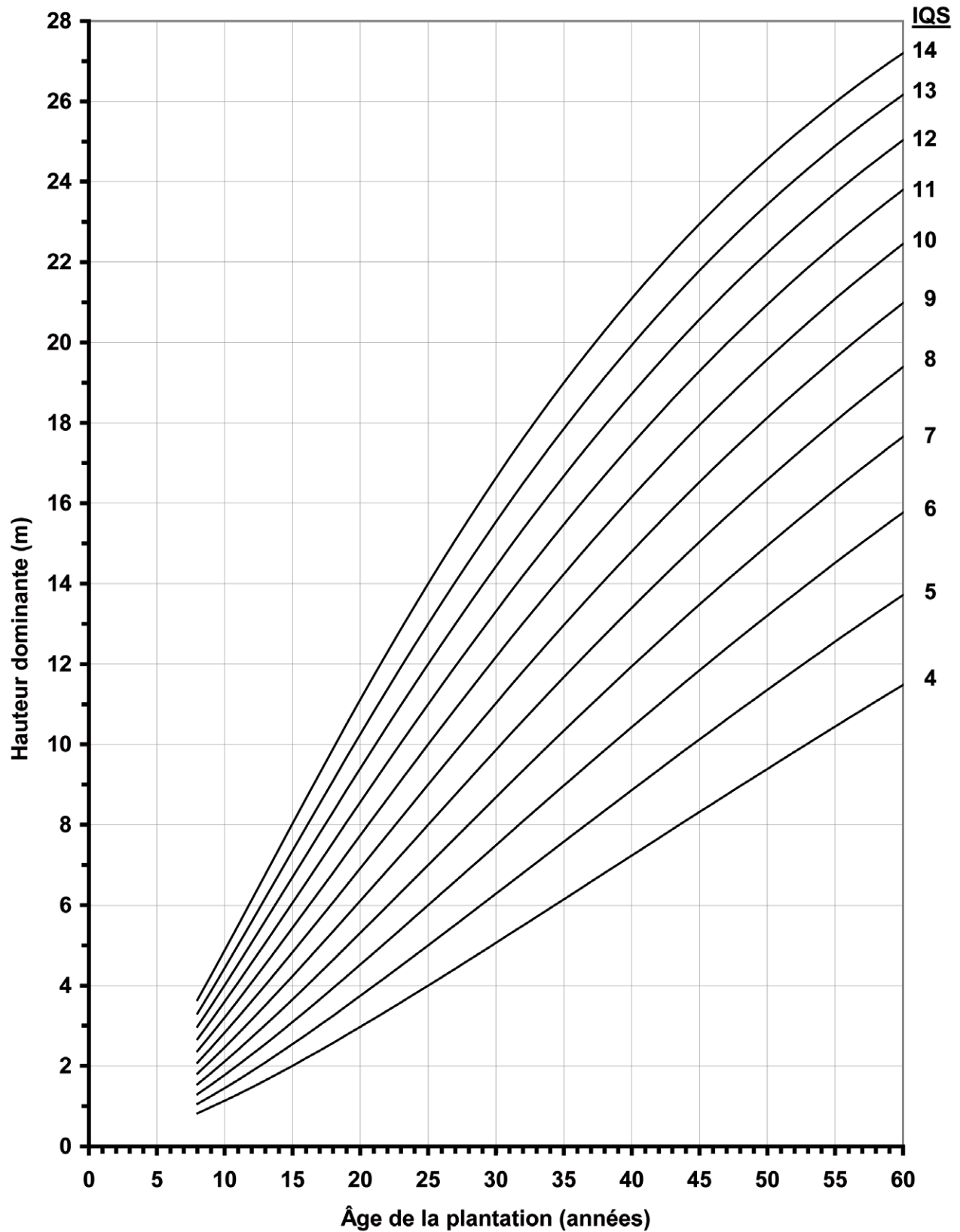
Figure 4. Hauteur dominante de l'épinette blanche en fonction de l'âge pour divers indices de qualité de station.
