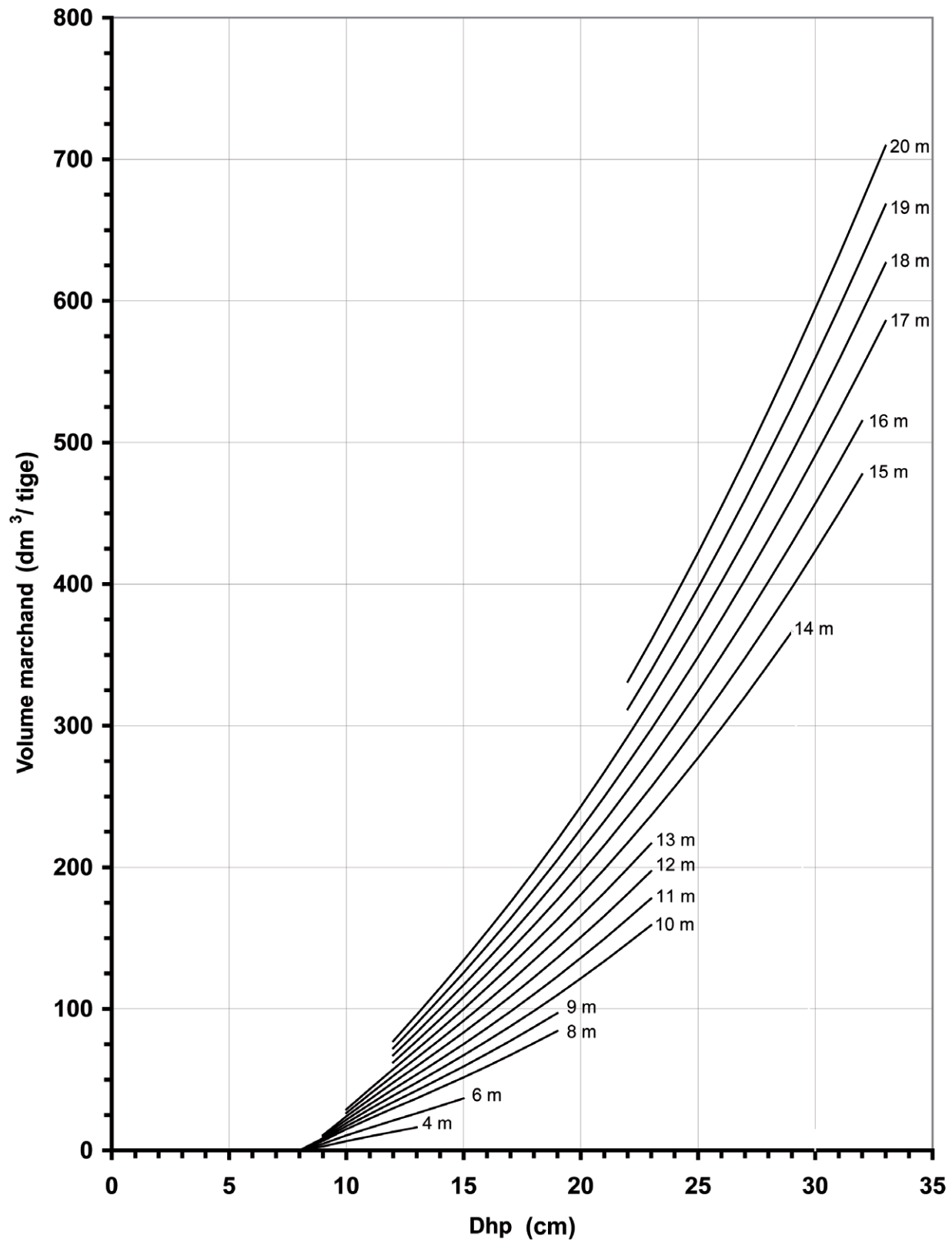
Figure 3. Volume marchand d'une tige d'épinette blanche en plantation en fonction du dhp et de la hauteur totale.
