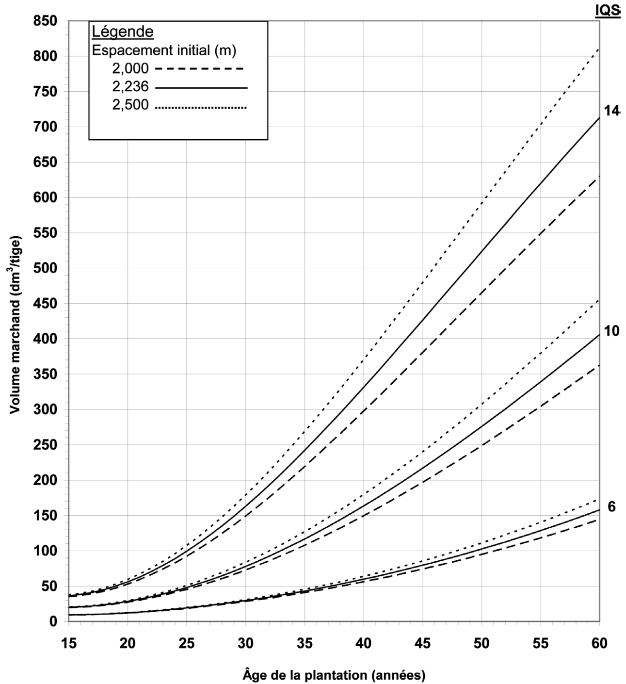
Figure 9. Volume marchand par tige estimé à partir des modèles des tables de rendement selon divers IQS et espacements initiaux, pour les plantations d'épinette blanche.
