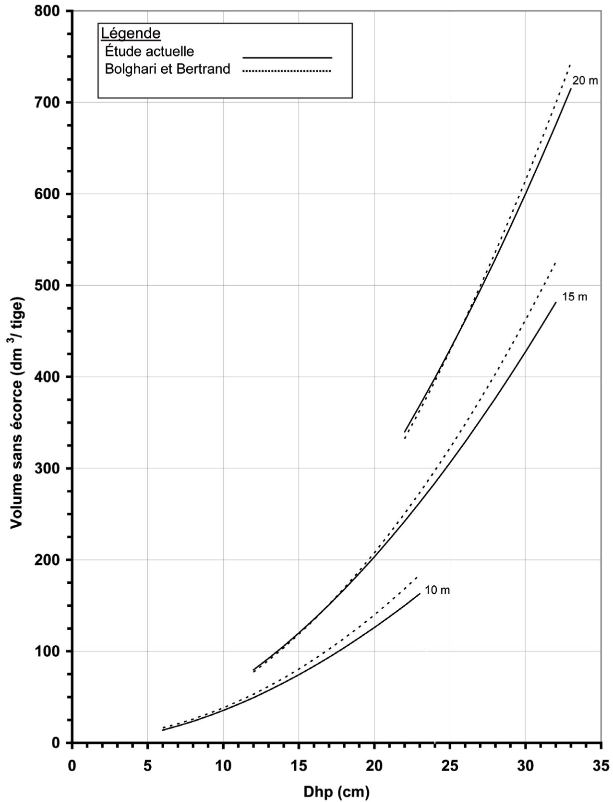
Figure 5. Comparaison du volume total sans écorce estimé par les tarifs de cubage de BOLGHARI et BERTRAND (1984) et celui de l'étude actuelle.
