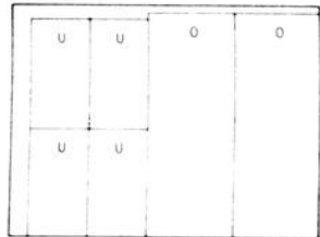
SCHEMA DE DEBITAGE morceau de contre-plaqué 32" x 42"
