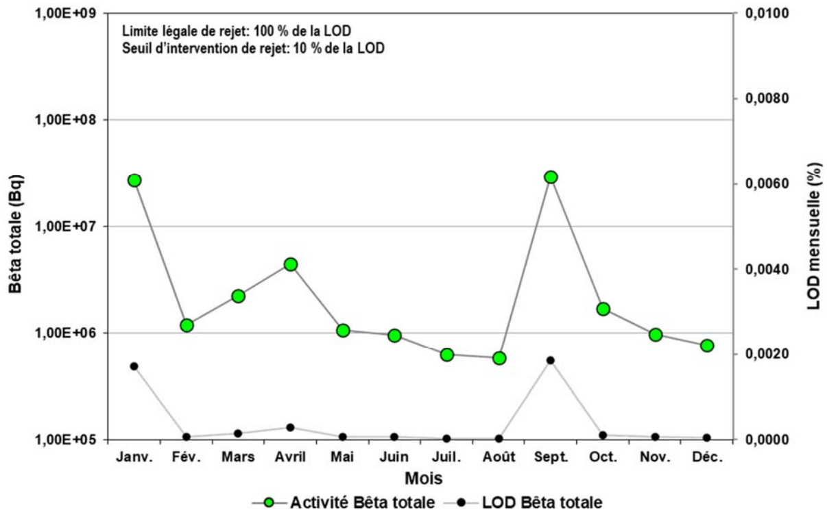
Figure 2-7 : Présence d'activité bêta totale aux effluents liquides de l'installation nucléaire de Gentilly-2, exprimée en % LOD et en activité sur une base mensuelle pour l'année 2021
