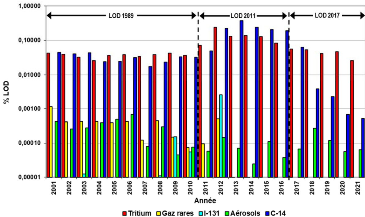
Figure 2-4 : Rejets radioactifs gazeux annuels de l'installation nucléaire de Gentilly-2 exprimés en % LOD pour la période 2001-2021
