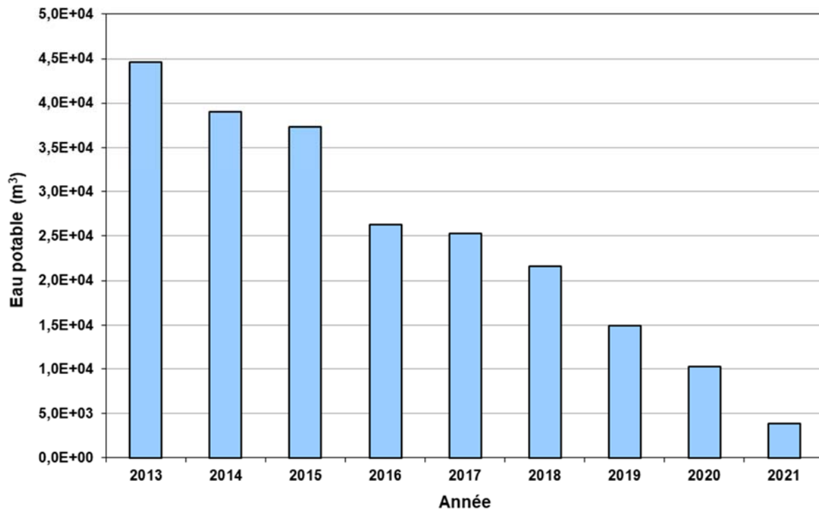
Figure 5-2 : Consommation d'eau potable aux installations de Gentilly-2 pour la période 2013-2021
