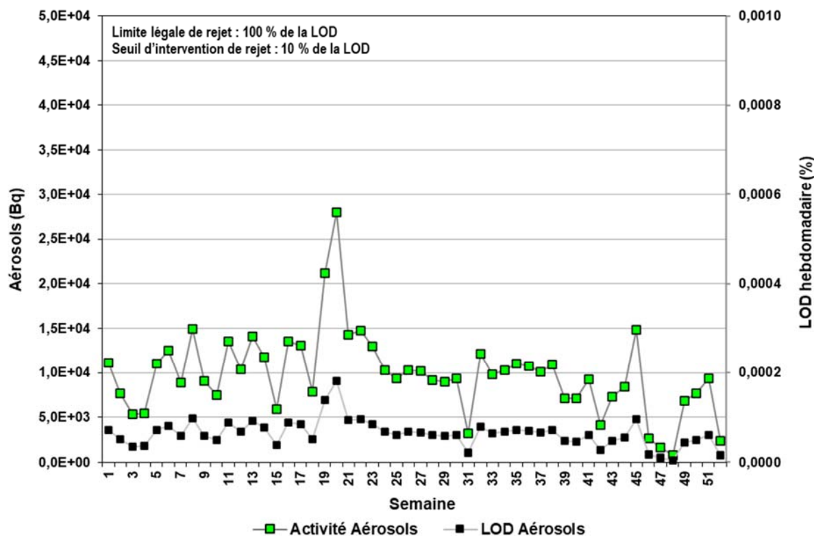
Figure 2-3 : Présence d'aérosols radioactifs aux rejets gazeux de l'installation nucléaire de Gentilly-2, exprimée en % LOD et en activité sur une base hebdomadaire pour l'année 2021
