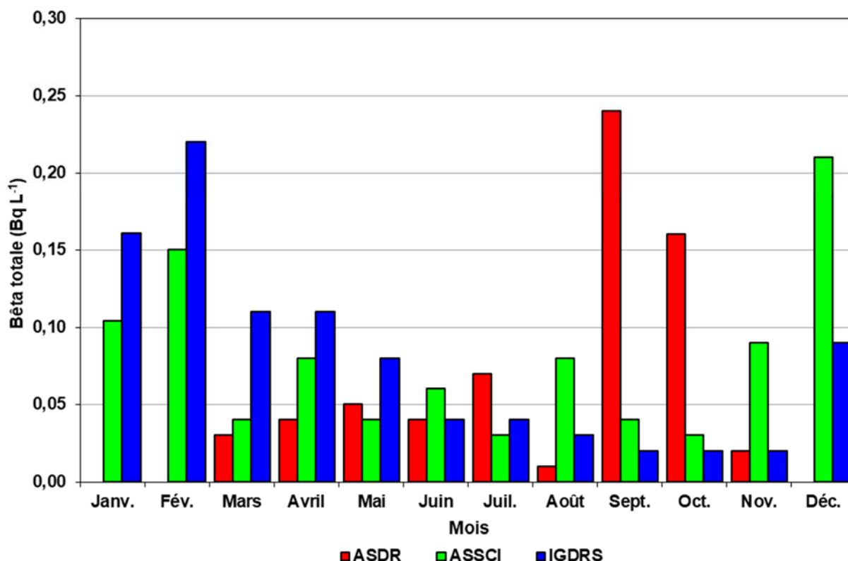
Figure 8-32 : Moyenne mensuelle de l'activité bêta totale dans l'eau de surface autour de l'ASDR, de l'ASSCI et de l'IGDRS pour l'année 2021
