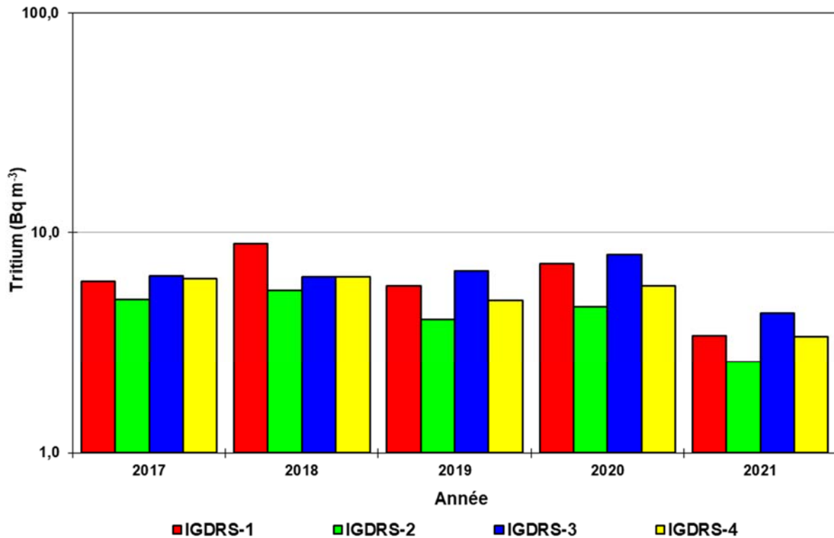
Figure 8-16 : Activité annuelle moyenne de tritium atmosphérique à l'IGDRS pour la période 2017-2021
