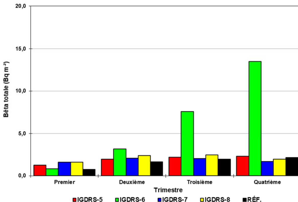
Figure 8-29 : Moyenne trimestrielle de l'activité bêta totale dans les précipitations aux stations IGDRS-5 à 8 et à la station de référence pour l'année 2021
