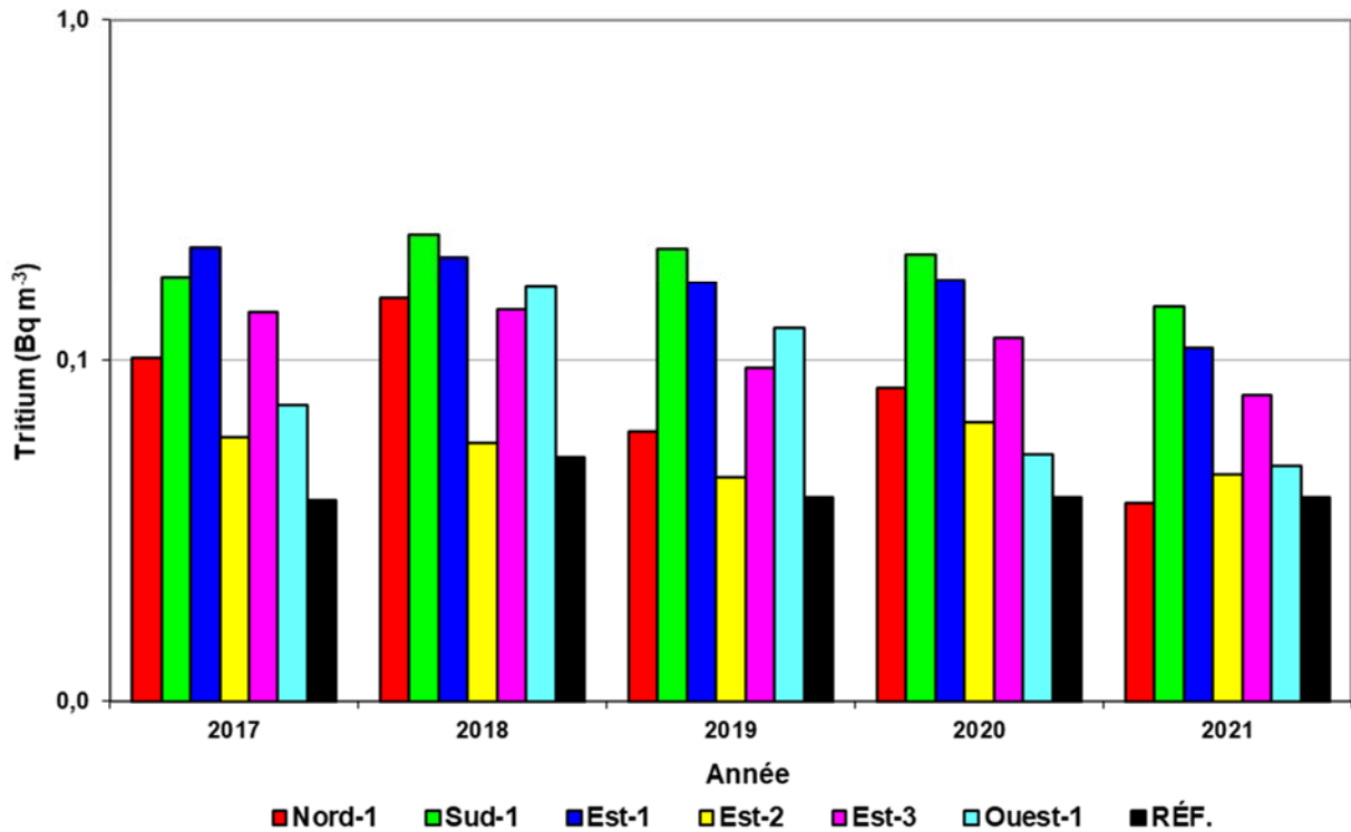
Figure 8-14 : Activité annuelle moyenne en tritium atmosphérique aux stations Nord-1, Sud-1, Est-1 à Est-3, Ouest-1 et à la station de référence pour la période 2017-2021
