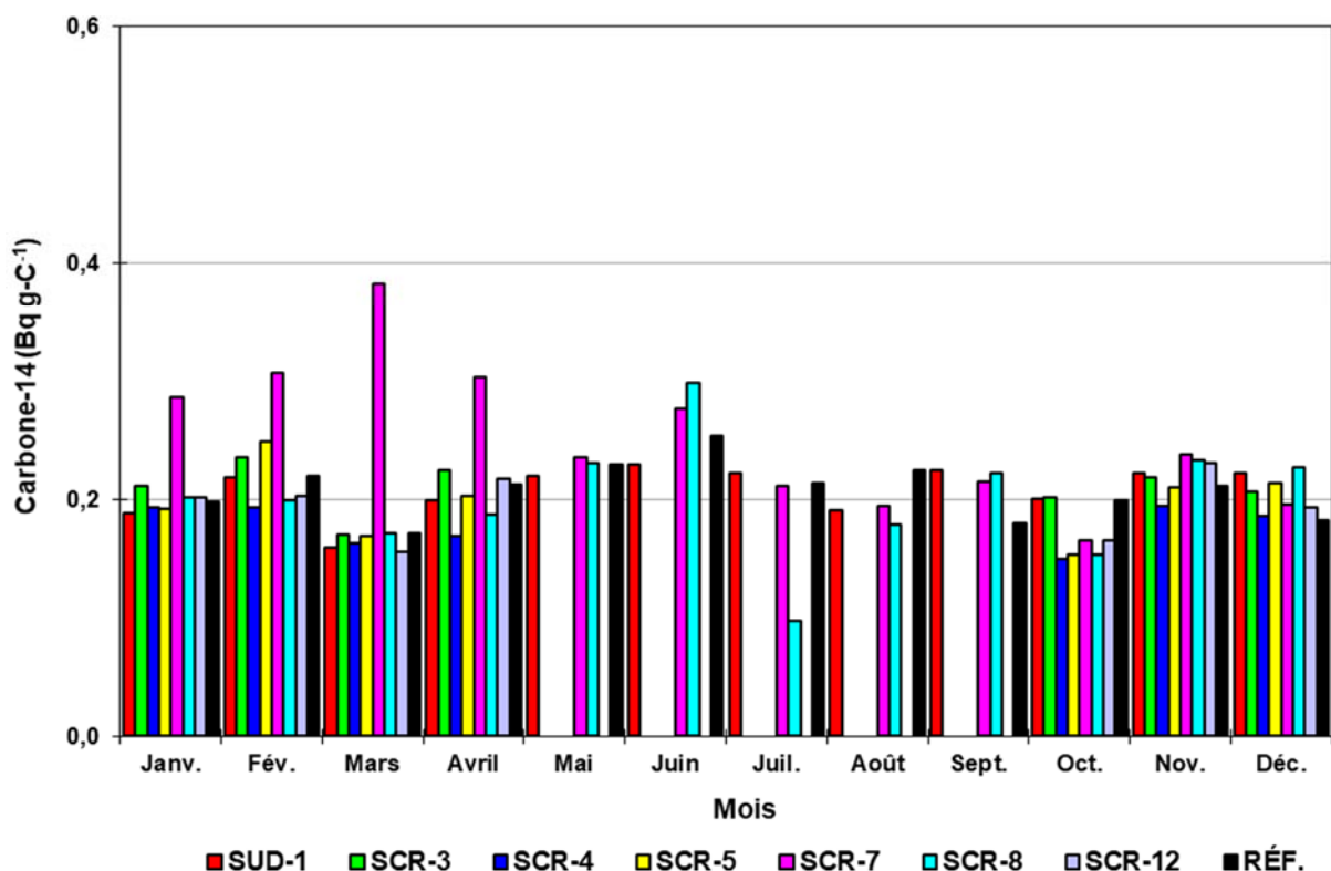
Figure 8-19 : Activité mensuelle en carbone-14 atmosphérique aux stations Sud-1, SCR-3 à SCR-5, SCR-7, SCR-8, SCR-12 (zone rapprochée) et à la station de référence pour l'année 2021
