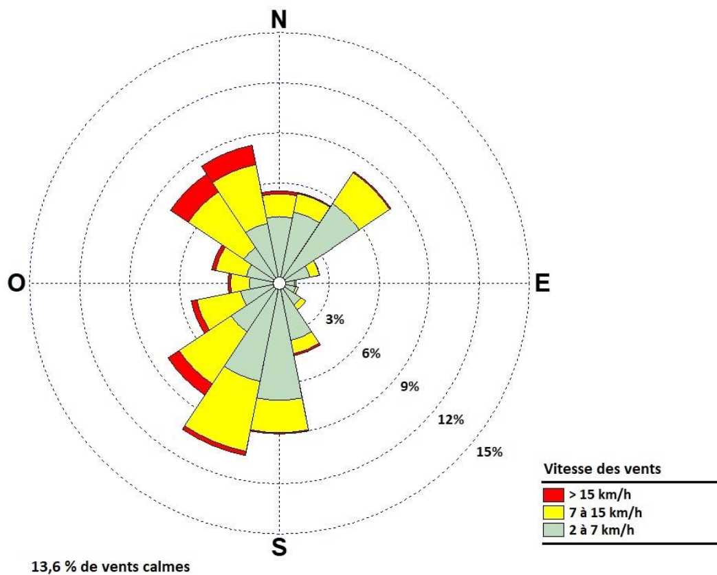
Figure 8-42 : Rose de l'origine des vents au site instrumenté du MELCC à Bécancour pour l'année 2021
