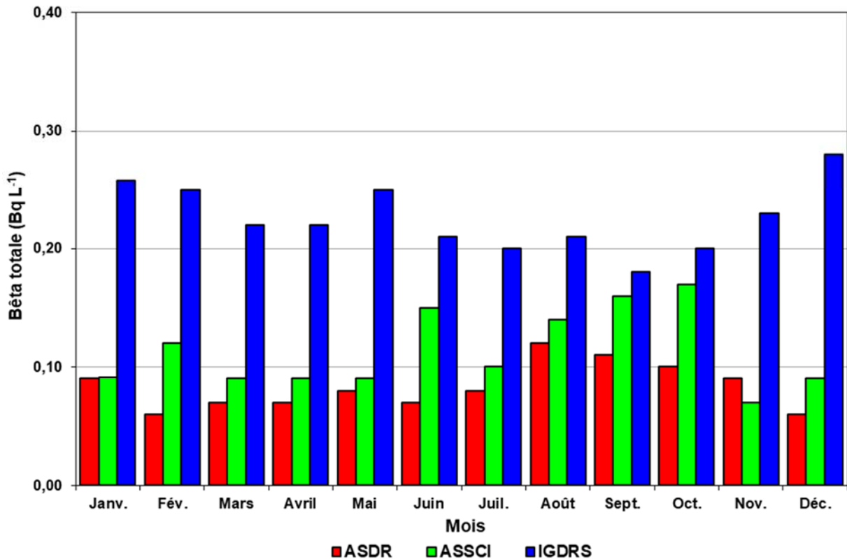
Figure 8-35 : Moyenne mensuelle de l'activité bêta totale dans l'eau d'infiltration autour de l'ASDR, de l'ASSCI et de l'IGDRS pour l'année 2021
