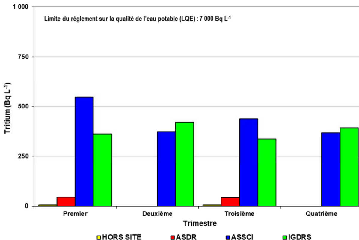
Figure 8-36 : Moyenne trimestrielle de l'activité en tritium dans l'eau souterraine de l'ASDR, de l'ASSCI, de l'IGDRS et hors site pour l'année 2021
