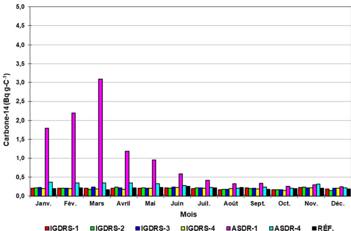
Figure 8-21 : Activité mensuelle en carbone-14 atmosphérique à l'IGDRS, à l'ASDR et à la station de référence pour l'année 2021
