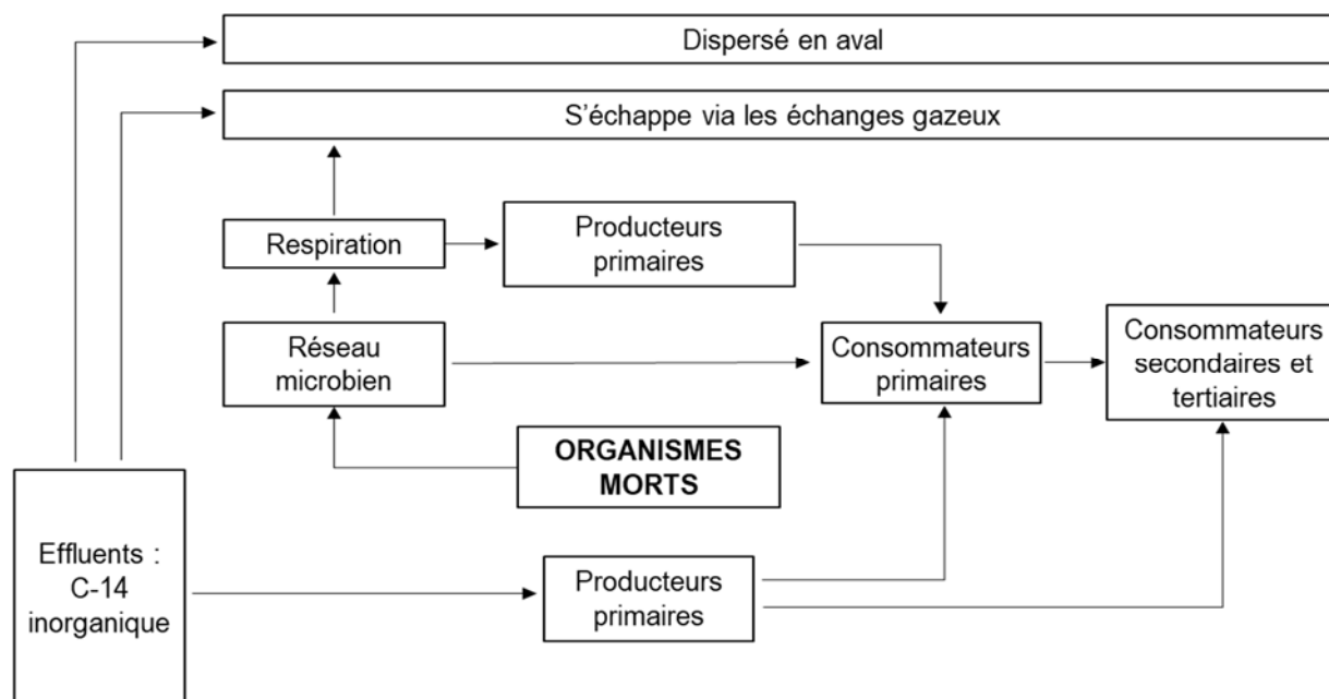
Figure 8-39 : Représentation simplifiée du flux de carbone-14 dans le milieu aquatique à proximité des installations de Gentilly-2
