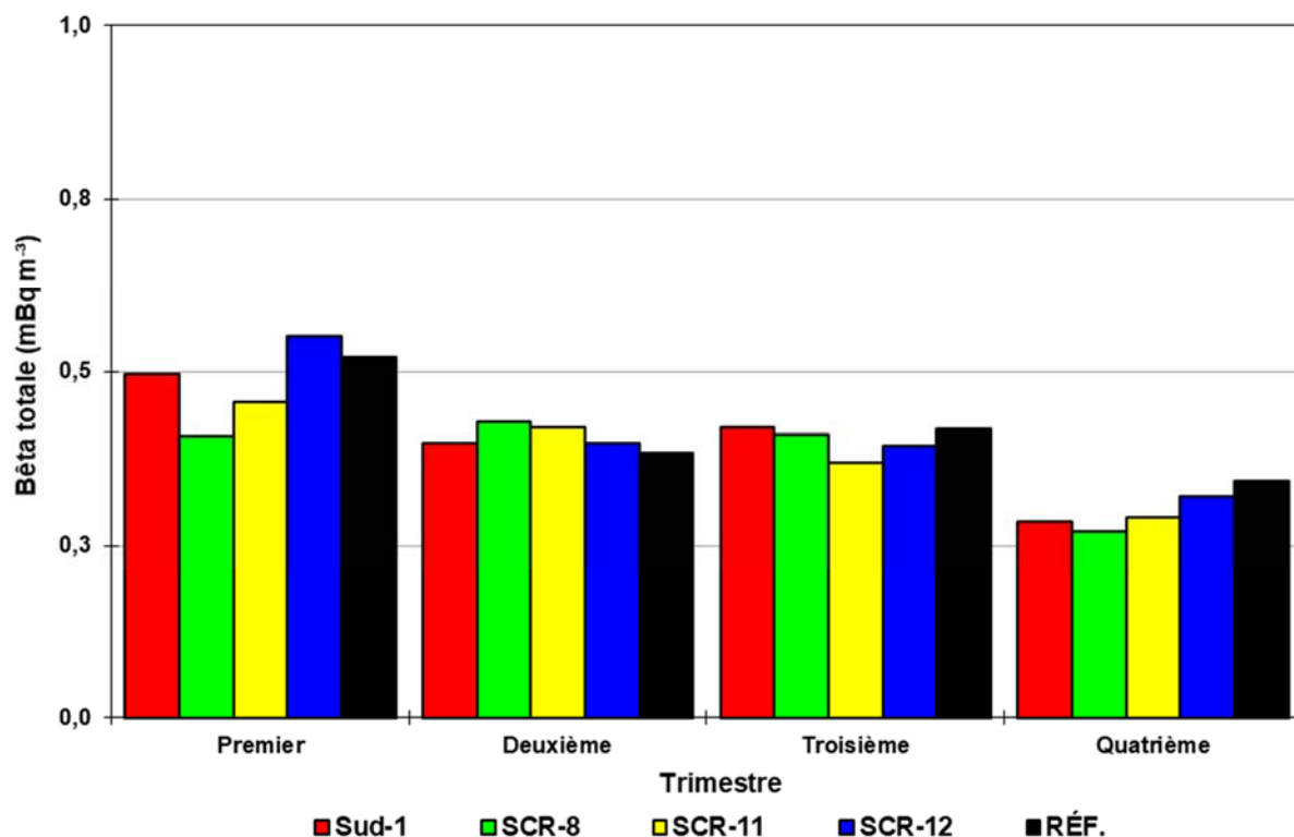
Figure 8-23 : Moyenne trimestrielle de l'activité bêta totale dans les aérosols prélevés aux stations Sud-1, SCR-8, SCR-11, SCR-12 et à la station de référence pour l'année 2021
