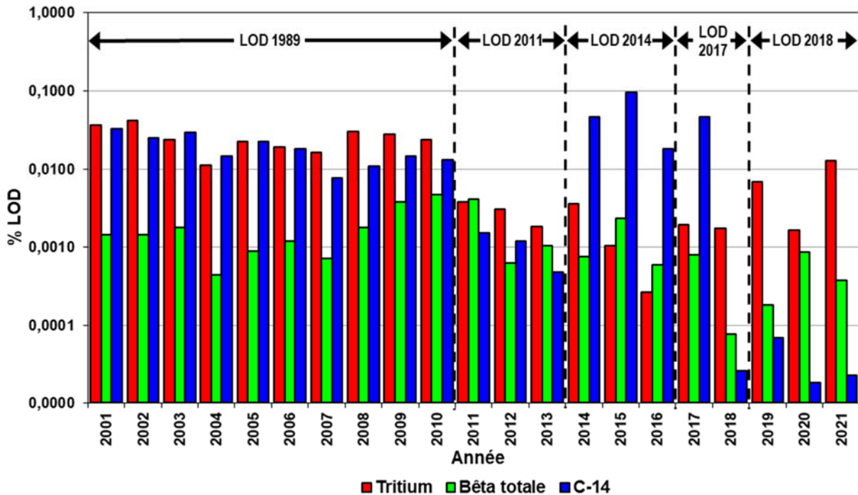
Figure 2-8 : Rejets radioactifs liquides annuels de l'installation nucléaire de Gentilly-2 exprimés en % LOD pour la période 2001-2021
