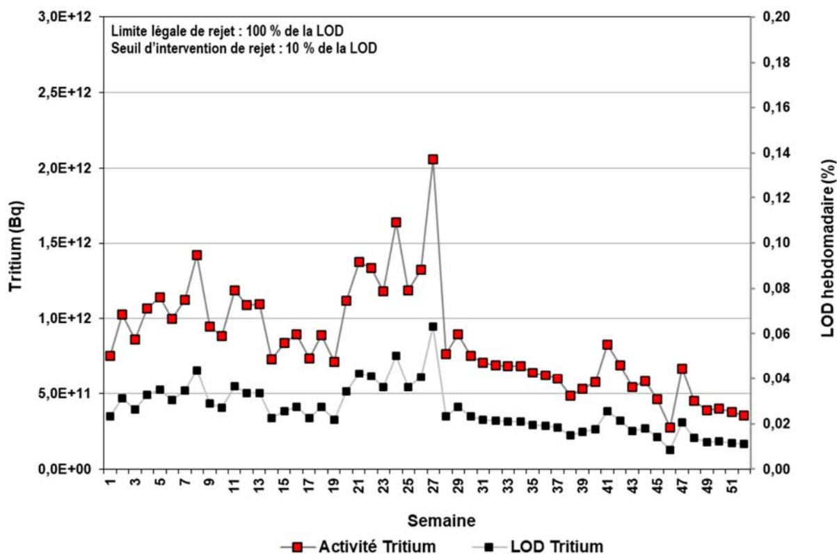
Figure 2-1 : Présence de tritium aux rejets gazeux de l'installation nucléaire de Gentilly-2, exprimée en % LOD et en activité sur une base hebdomadaire pour l'année 2021
