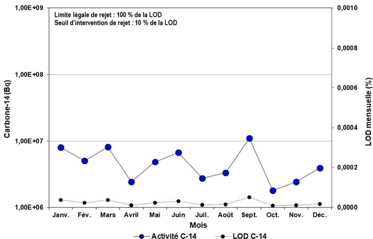
Figure 2-6 : Présence de carbone-14 aux effluents liquides de l'installation nucléaire de Gentilly-2, exprimée en % LOD et en activité sur une base mensuelle pour l'année 2021
