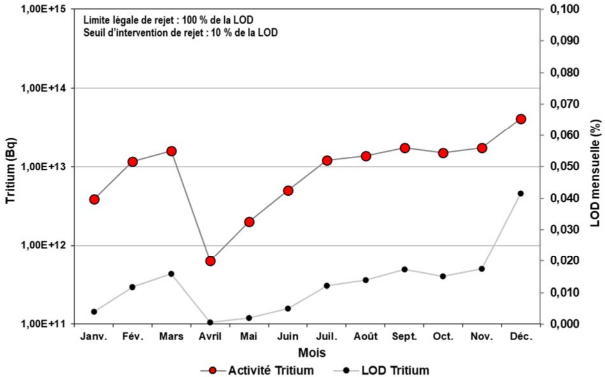
Figure 2-5 : Présence de tritium aux effluents liquides de l'installation nucléaire de Gentilly-2, exprimée en % LOD et en activité sur une base mensuelle pour l'année 2021
