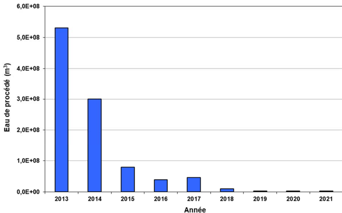
Figure 5-1 : Consommation d'eau de procédé aux installations de Gentilly-2 pour la période 2013-2021
