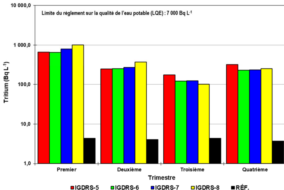
Figure 8-28 : Moyenne trimestrielle de l'activité en tritium dans les précipitations aux stations IGDRS-5 à 8 et à la station de référence pour l'année 2021
