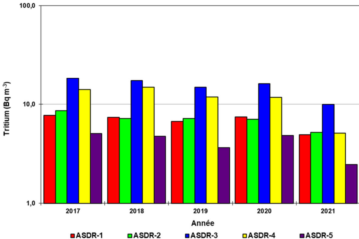
Figure 8-18 : Activité annuelle moyenne de tritium atmosphérique à l'ASDR pour la période 2017-2021
