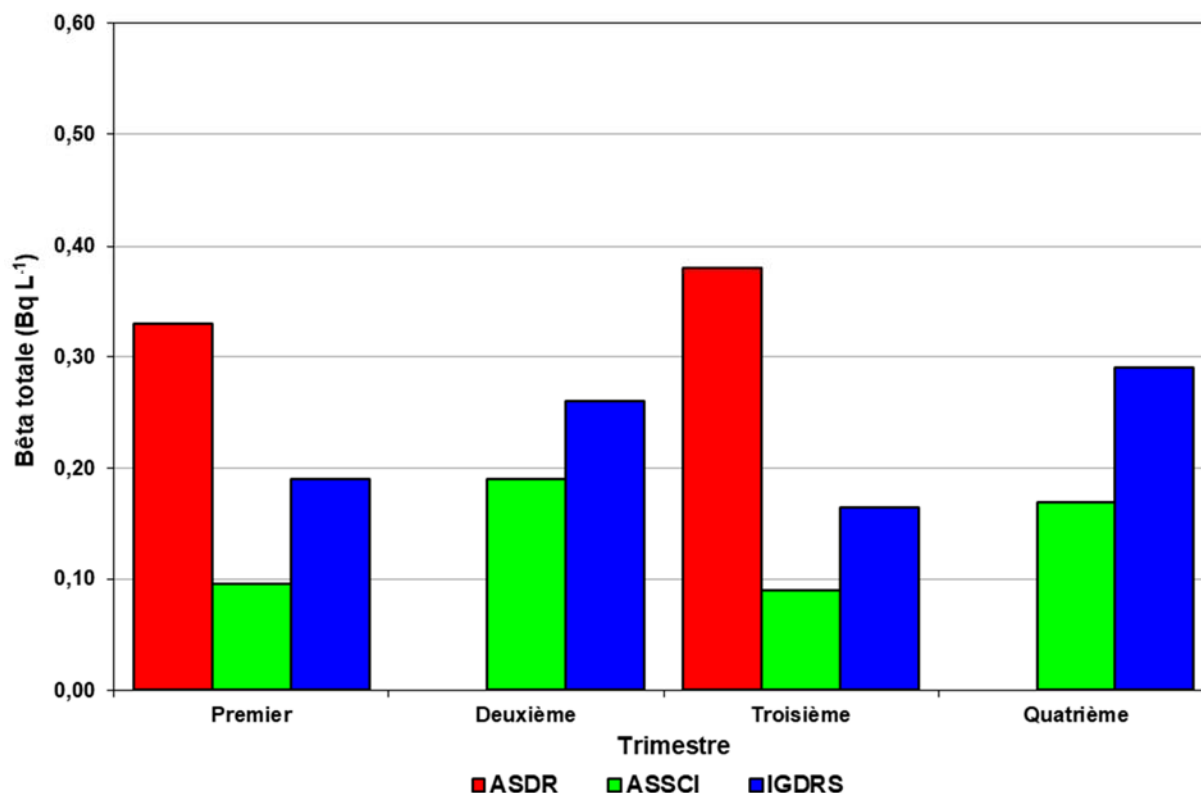
Figure 8-38 : Moyenne trimestrielle de l'activité bêta totale dans l'eau souterraine autour de l'ASDR, de l'ASSCI et de l'IGDRS pour l'année 2021
