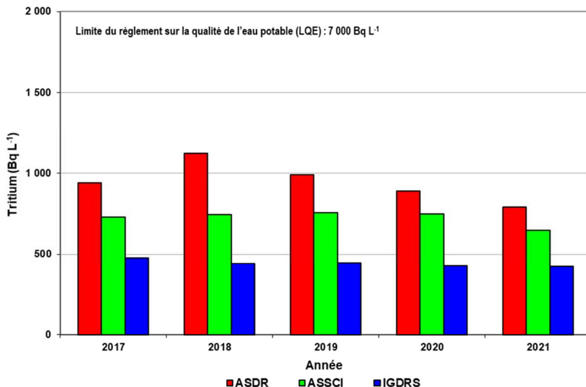
Figure 8-34 : Moyenne annuelle de l'activité en tritium dans l'eau d'infiltration autour de l'ASDR, de l'ASSCI et de l'IGDRS pour la période 2017-2021
