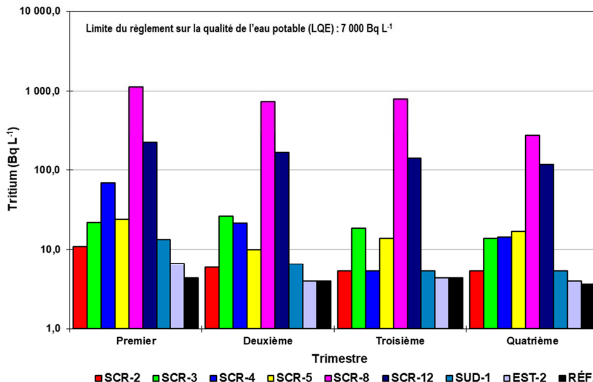
Figure 8-26 : Moyenne trimestrielle de l'activité en tritium dans les précipitations aux stations SCR-2 à SCR-5, SCR-8, SCR-12, Sud-1, Est-2 et de référence pour l'année 2021
