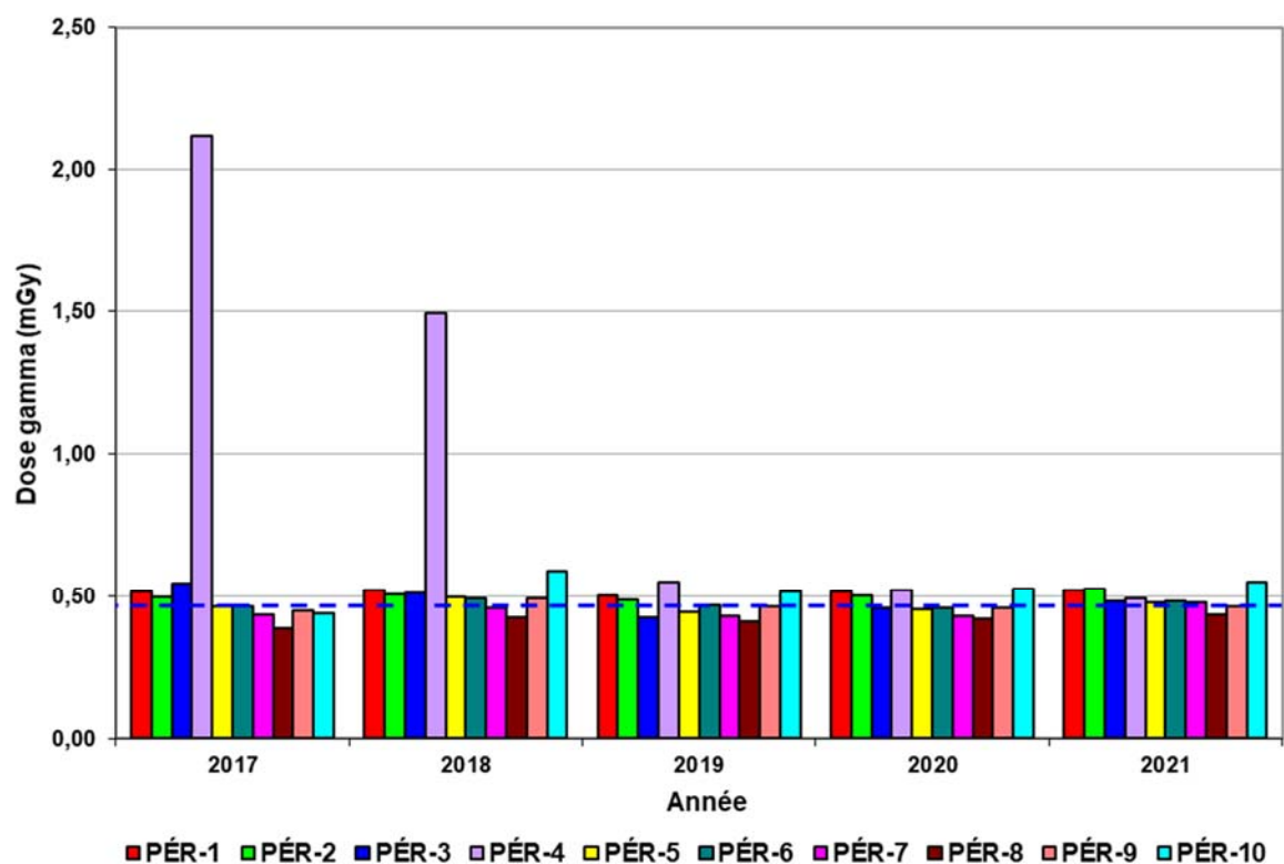
Figure 8-4 : Dose annuelle gamma au périmètre sécurisé de l'installation pour la période 2017-2021
