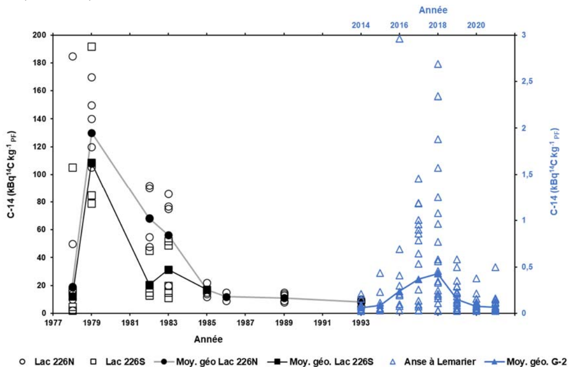
Figure 8-41 : Évolution temporelle du carbone-14 dans les poissons du lac 226 (1978 à 1993) et de l'anse à Lemarier (2014 à 2021)
