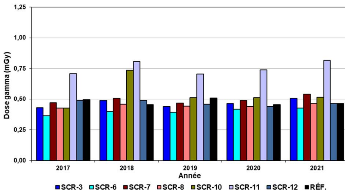
Figure 8-2 : Dose annuelle gamma aux stations de contrôle SCR-3, 6, 7, 8, 10, 11 et 12 (zone rapprochée) et à la station de référence pour la période 2017-2021
