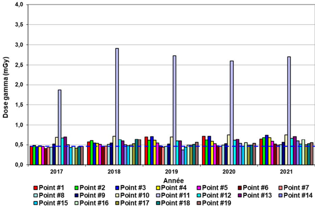
Figure 8-8 : Dose annuelle gamma à la clôture de l'IGDRS pour la période 2017-2021
