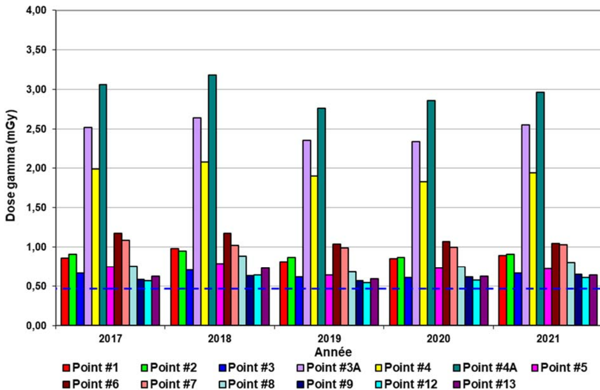
Figure 8-10 : Dose annuelle gamma à la clôture de l'ASSCI pour la période 2017-2021
