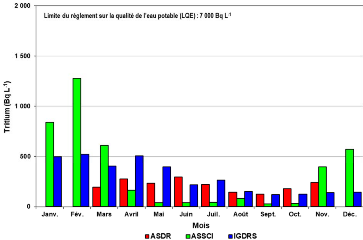
Figure 8-30 : Moyenne mensuelle de l'activité en tritium dans l'eau de surface autour de l'ASDR, de l'ASSCI et de l'IGDRS pour l'année 2021
