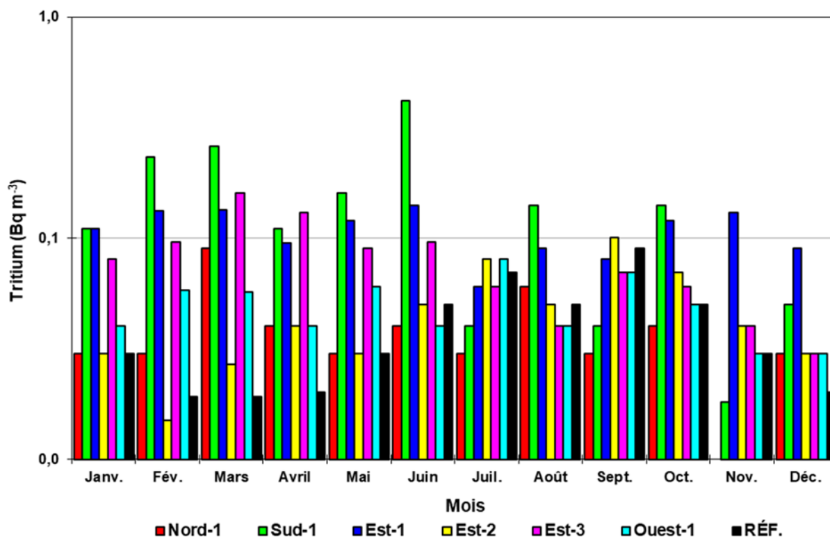
Figure 8-13 : Activité mensuelle en tritium atmosphérique aux stations Nord-1, Sud-1, Est-1 à Est-3, Ouest-1 et à la station de référence pour l'année 2021
