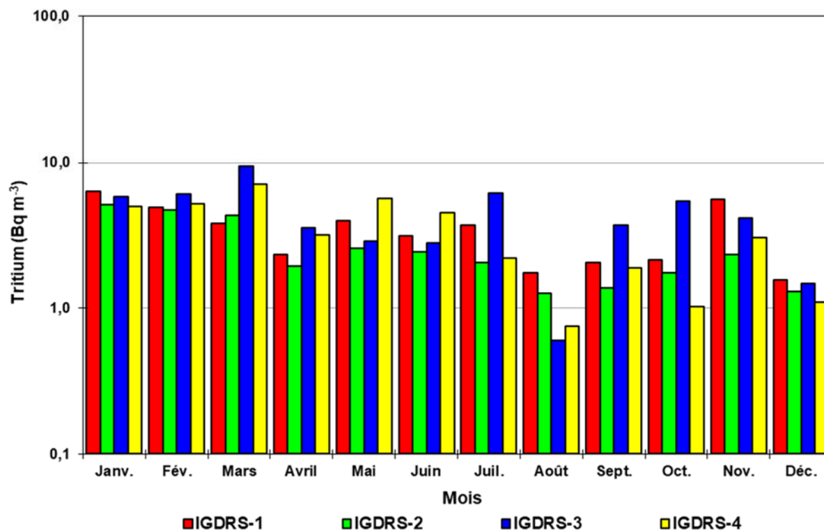
Figure 8-15 : Activité mensuelle en tritium atmosphérique à l'IGDRS pour l'année 2021
