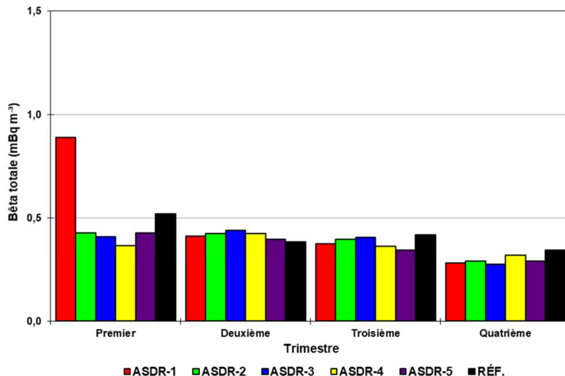
Figure 8-25 : Moyenne trimestrielle de l'activité bêta totale dans les aérosols prélevés à l'ASDR et à la station de référence pour l'année 2021
