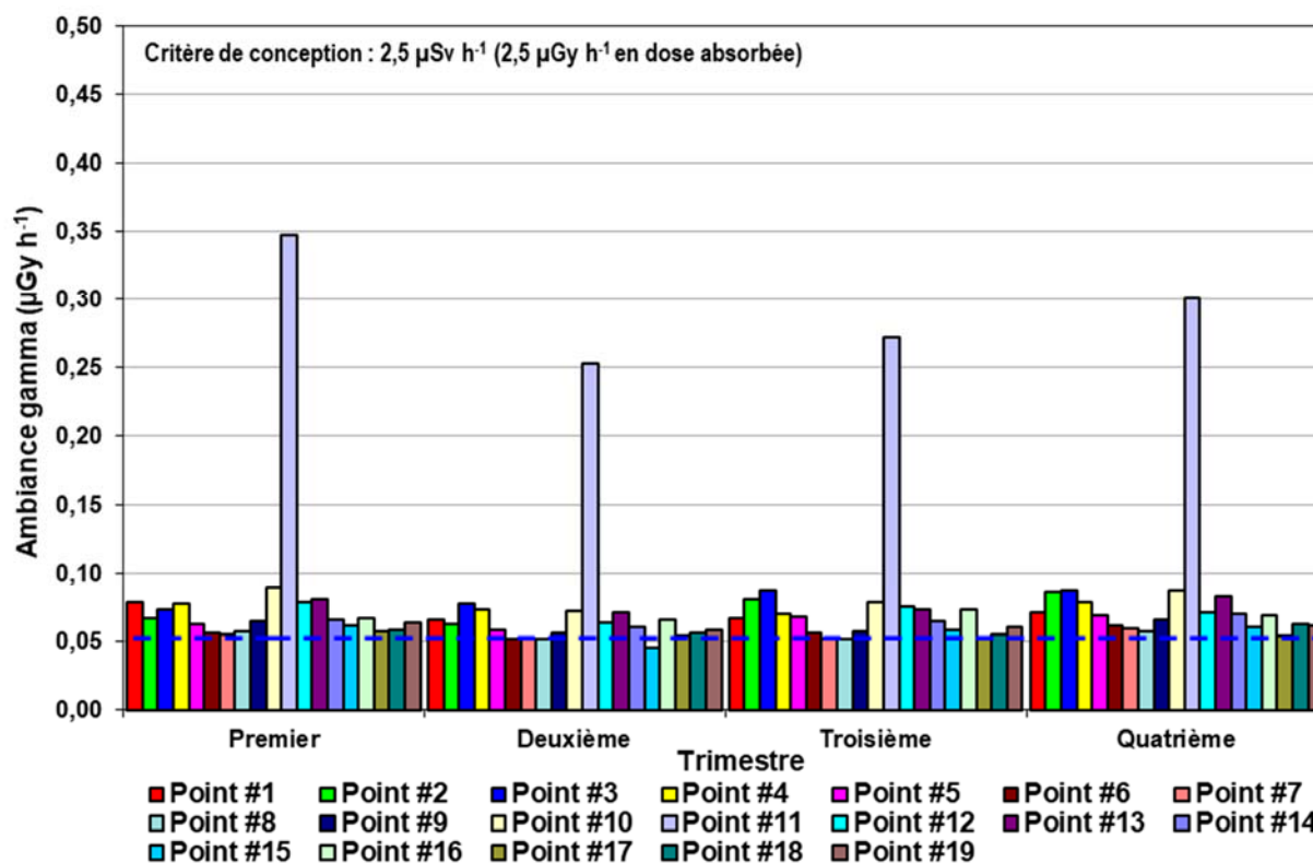
Figure 8-7 : Ambiance gamma trimestrielle à la clôture de l'IGDRS pour l'année 2021
