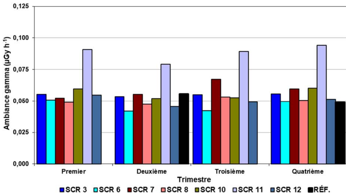
Figure 8-1 : Ambiance gamma trimestrielle aux stations de contrôle SCR-3, 6, 7, 8, 10, 11 et 12 (zone rapprochée) et à la station de référence pour l'année 2021
