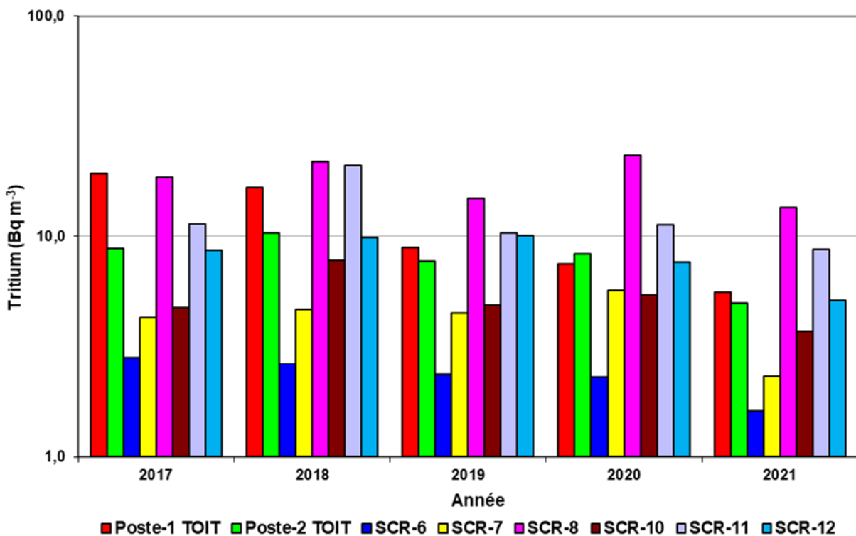
Figure 8-12 : Activité annuelle moyenne en tritium atmosphérique aux stations Poste-1, Poste-2, SCR-6 à SCR-8 et SCR-10 à SCR-12 (zone d'exclusion) pour la période 2017-2021
