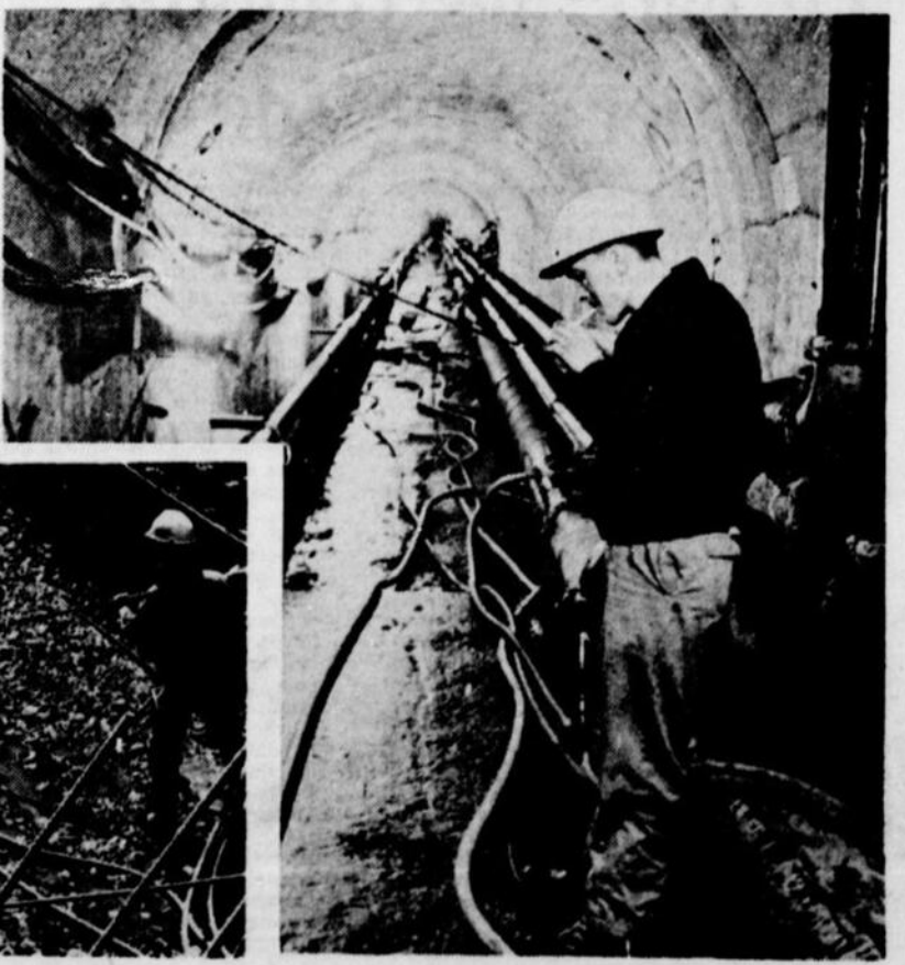
Ce tunnel, il est à l'intérieur de l'énorme masse de béton. Au-dessus du tunnel, on lave le ciment à la vapeur avant une nouvelle coulée.
