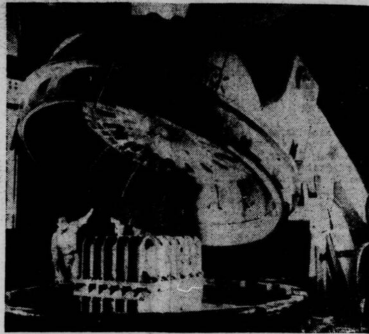
Cet appareil est employé pour vulcaniser les réservoirs de gazoline sur les avions de guerre. Le moule contenant le réservoir à fermer est placé dans l'appareil et le couvercle est rabattu avant qu'on y fasse arriver la chaleur. Ces réservoirs éliminent le danger des feux de gazoline causés par des bombes incendiaires ou les balles.
