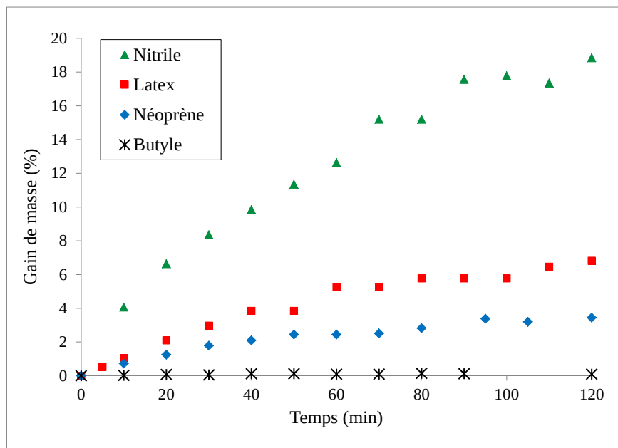
Figure 29 - Variation du gain de masse du nitrile, du latex, du néoprène et du butyle en fonction du temps d'immersion dans la solution colloïdale de \text{TiO}_2 dans l'eau
