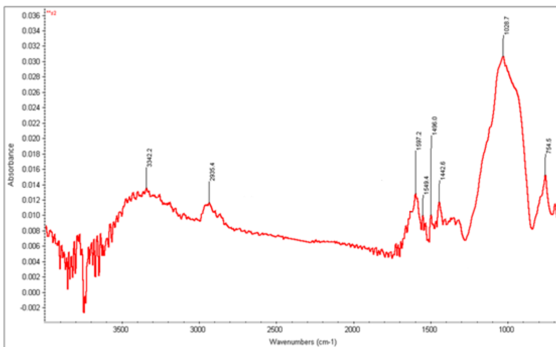
Figure 33 – Spectre FT-IR correspondant aux résidus de gonflement du néoprène dans l'EG pendant 7 jours
