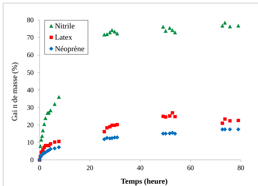
Figure 30 - Variation du gain de masse du nitrile, du latex et du néoprène pour des longs temps d'immersion dans la solution colloïdale de \text{TiO}_2 dans l'eau
