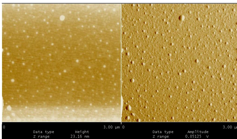
Figure 43 – Image AFM à une échelle de 3 μm d'une solution d'échantillonnage dans l'eau pure centrifugée sur un substrat de mica correspondant à un échantillon de nitrile soumis pendant 7 heures à des déformations dynamiques biaxiales (50%) et à de la poudre de TiO 2
