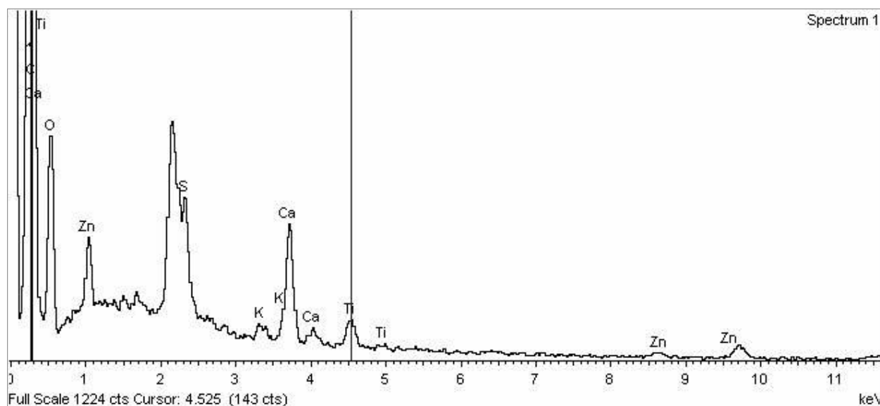
Figure 18 – Exemple de spectre EDS de la surface externe du gant en nitrile
