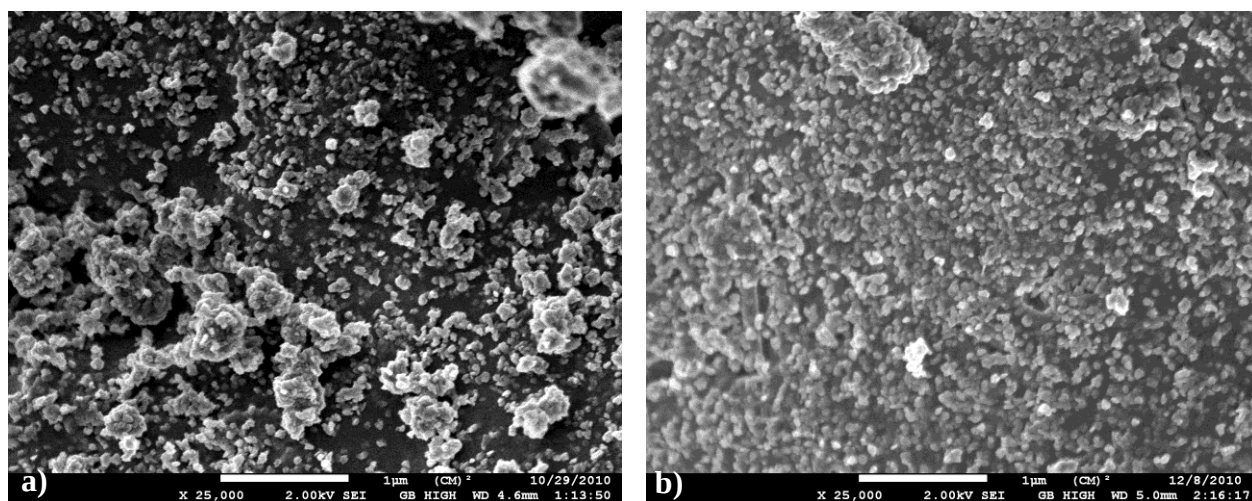
Figure 24 – Clichés au MEB-FEG de la surface d'échantillons en néoprène exposés à de la poudre de la \text{TiO}_2 conjointement avec des déformations dynamiques biaxiales de 50% pendant des durées de a) 1h 30 et b) 7h
