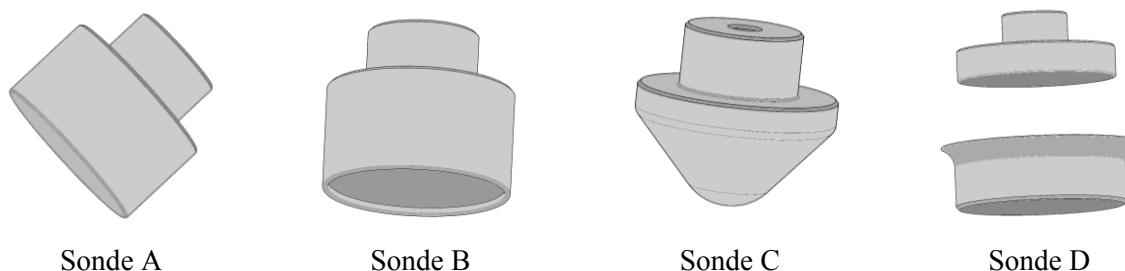
Figure 4 - Géométries disponibles pour l'extrémité de la sonde de déformation
