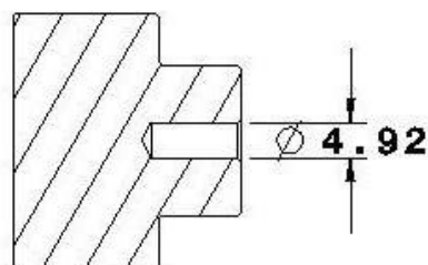
Coupe K-K Echelle : 1:1
