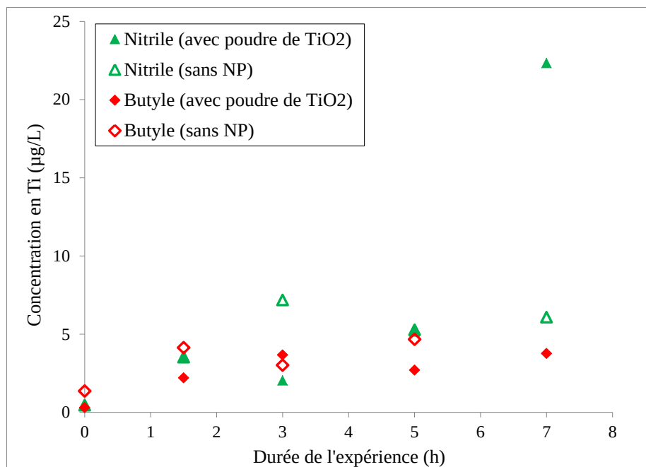
Figure 42 – Mesures par ICP-MS de la quantité de titane dans la solution d'échantillonnage en fonction de la durée de l'expérience pour le nitrile et le butyle exposés ou non à de la poudre de \text{TiO}_2 en plus des sollicitations dynamiques biaxiales
