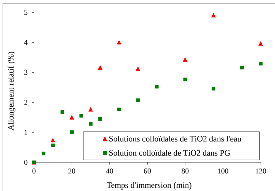
Figure 32 – Variation de l'allongement relatif du nitrile (orientation transverse) en fonction du temps d'immersion dans les solutions colloïdales de \text{TiO}_2 dans l'eau et dans le PG
