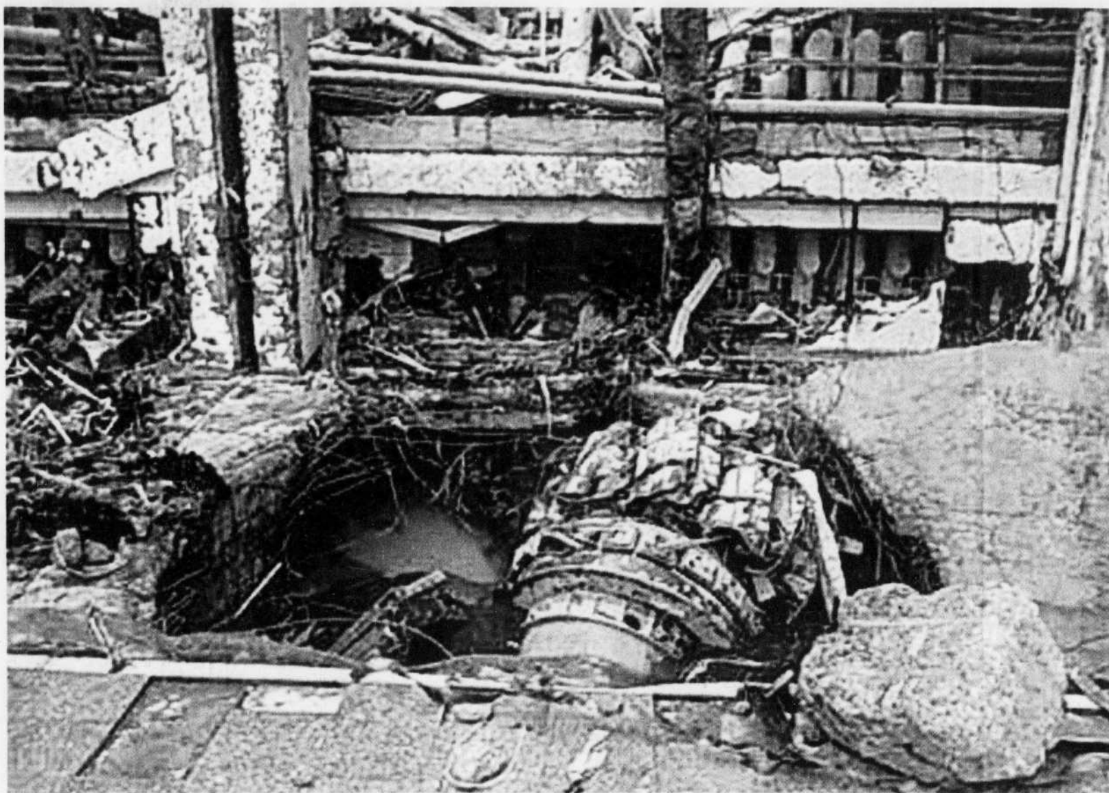
Une partie très endommagée de la centrale hydroélectrique de Saïano Chouchenskaïa, en Sibérie, photographiée par les services d'urgence russes.
