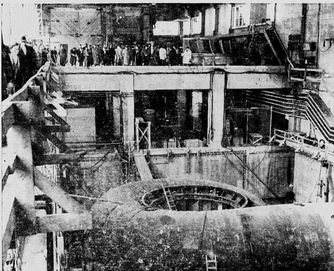
Les visiteurs regardent ici le colimaçon géant que représente la bache spirale à l'intérieur de laquelle sera plus tard installée la turbine qu'on voit à l'étage supérieur à la droite de la photo. C'est par la bache spirale que l'eau vient actionner la turbine après avoir fait une chute de 386 pieds.
