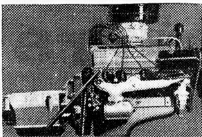
MOTEUR "ROCKET" DE 160 CVI —L'étonnant "Quadri-Jet", le nouveau carburateur révolutionnaire d'Oldsmobile, et un nouveau mécanisme de soupapes à haute élévation ont ajouté 25 CV de plus au célèbre moteur "Rocket" à haute compression.
