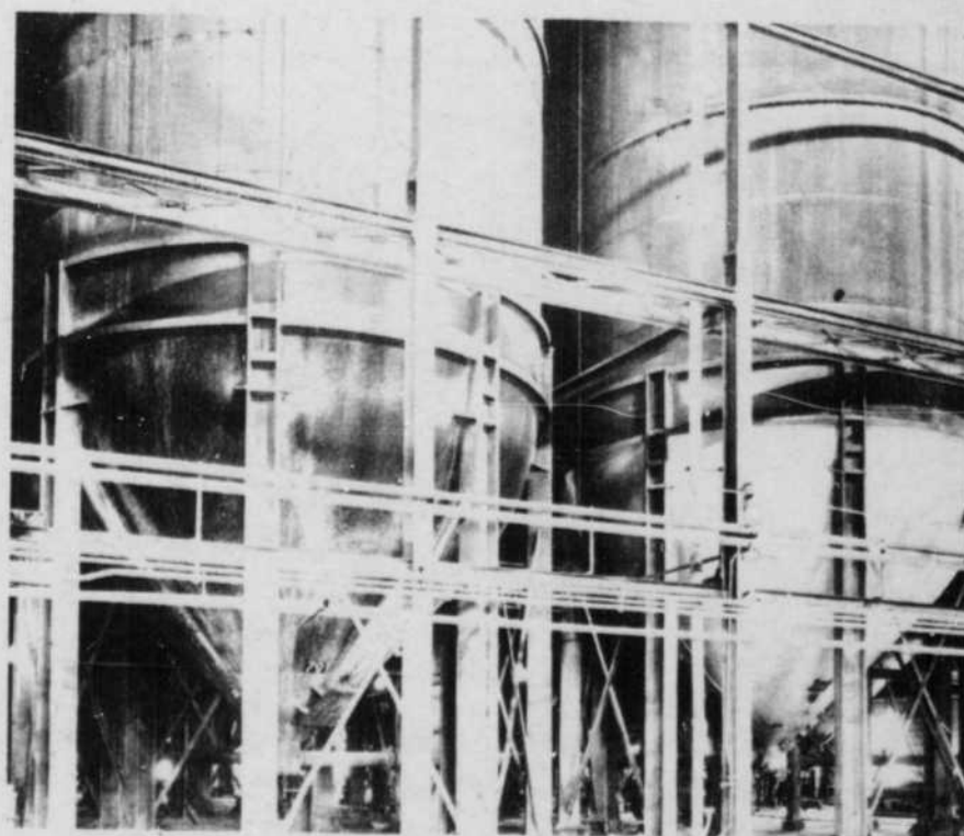
Vue de décomposeurs (précipitateurs) à l'usine de minerai No 2. La photographie ne nous permet pas de mesurer la hauteur de ces cuves. De fait, elles atteignent près de 80 pieds de hauteur.
