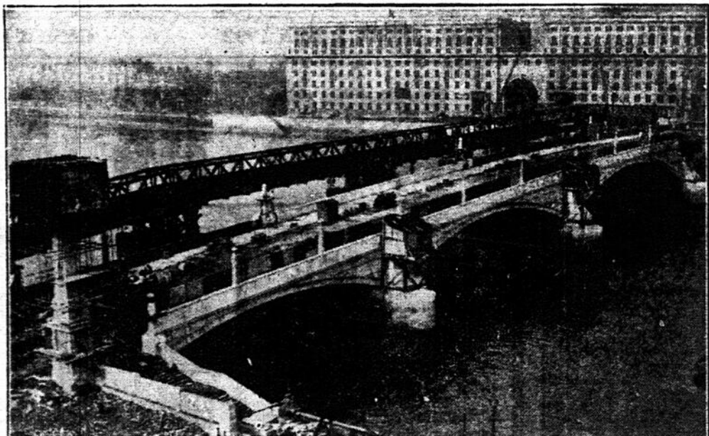
L'ELEGANCE PEUT S'ALLIER A LA MASSE:—Voici le nouveau pont Lambeth, jété au-dessus de la Tamise, à Londres. Ce pont tout en béton armé est des plus élégants. Au sommet de la photo, à droite, on voit la Thames House.
