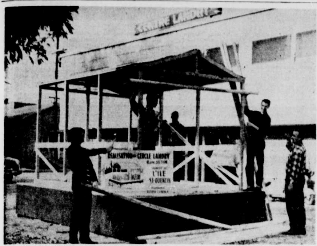
Le Centre Landry fera don d'un kiosque flottant au comité de l'île Saint-Quentin pour assurer une plus grande sécurité aux baigneurs. Le kiosque a été construit par un groupe de membres du centre dirigé par M. Jean Pelletier. On en voit quelques-uns à l'oeuvre sur la photo ci-dessus.
