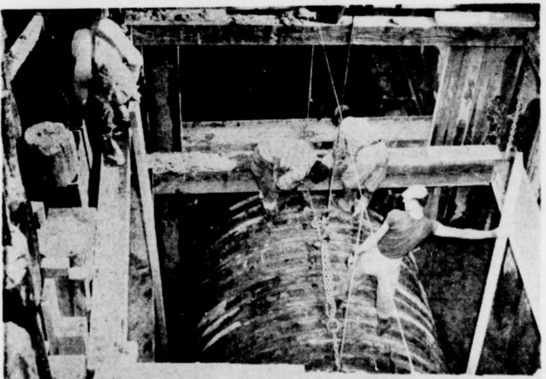
LA PREMIERE FEUILLE de l'enveloppe d'acier dans laquelle on glissera le tuyau d'égout de la rue Vézina a été mise en place, hier après-midi. L'immense pièce circulaire a été déposée par une grue mécanique au fond de la large tranchée qui traverse le chemin de fer du Pacifique Canadien. La photo ci-dessus montre bien l'envergure des travaux qui se déroulent dans un sol argileux et détrempé à l'excès.
