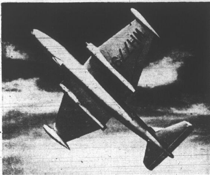
AVION SOUMIS A UN DUR ENTRAINEMENT — Un avion réacté "Canberra P.R.-7", semblable à celui illustré ci-haut, vient d'être soumis à un très dur entraînement par les autorités britanniques. En 25 jours, il fut dans les airs pendant 300 heures et couvrit une distance de quelque 156,000 milles. Des équipages se remplaçaient à tour de rôle pour cette épreuve faite à une altitude de 40,000 pieds.
