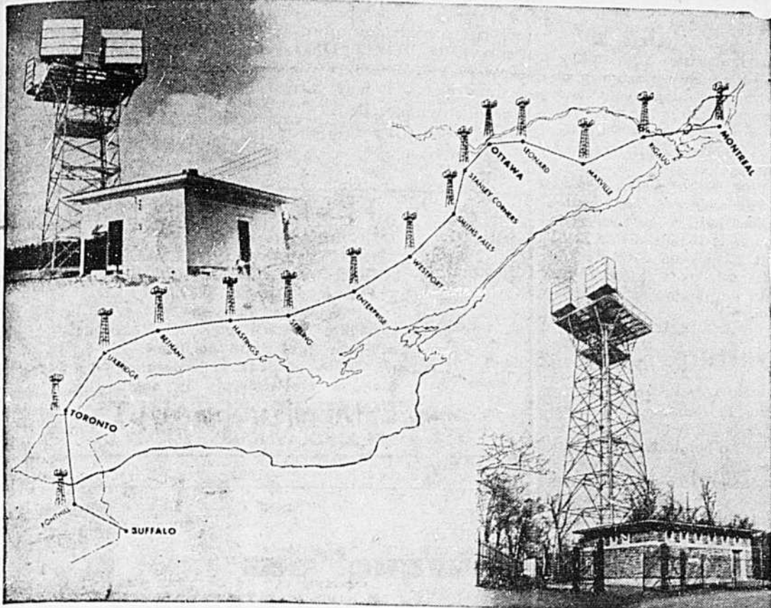
Carte du réseau de télévision de Radio-Canada avec ses relais à ondes micrométriques qui ont été érigés par la Compagnie de téléphone Bell. En bas, à droite, le pylône terminus de Montréal, qui a été érigé sur le mont Royal. On aperçoit à l'arrière-plan l'antenne de CBFT. En haut, à gauche, l'une des 13 stations de relais entre Montréal, Ottawa et Toronto.
