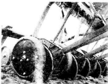
Les ouvre-sillons en V parfait facultatifs sont munis de roues jaugeuses de chaque côté des lames à double disque. Ils forment un sillon en V qui retient les semences à la profondeur choisie.
