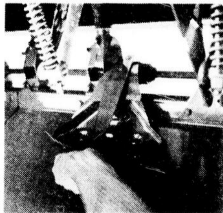
Ce levier permet de régler l'arbre d'alimentation pour mesurer de grandes ou de petites quantités de graines de semence.
