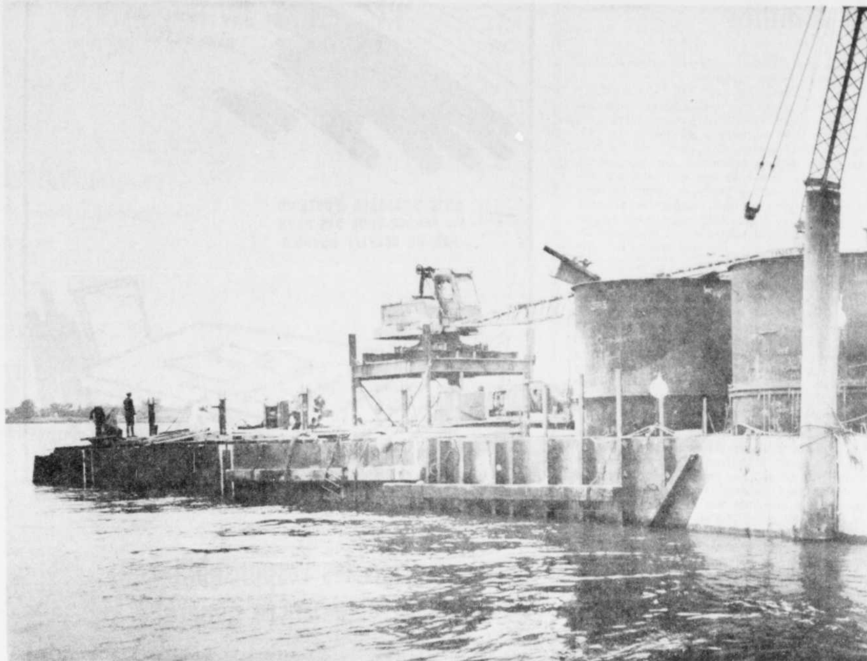
CETTE PHOTOGRAPHIE, prise à l'extérieur du caisson N-2, indique de façon excellente que la construction d'un batardeau autour de trois des quatre côtés du caisson a été complétée, afin de retenir les eaux du fleuve St-Laurent. Les employés de la Dufresne-McNamara s'affairent depuis plusieurs semaines à retirer les nombreux débris qui se sont accumulés à l'intérieur du caisson par suite de
