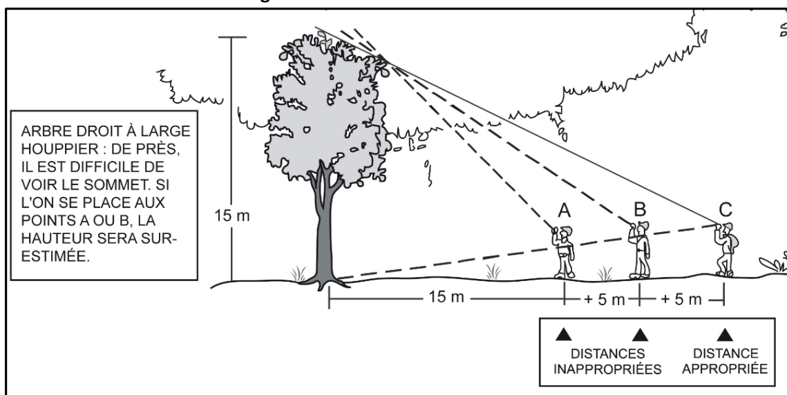
Figure 34 Mesure de hauteur d'arbre
