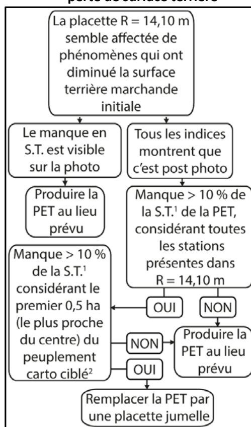
Figure 2 Évaluation de l'emplacement : perte de surface terrière
