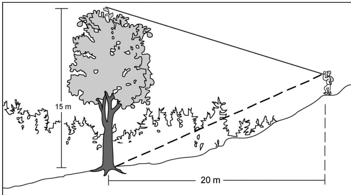
Figure 36 Mesure de hauteur d'arbre (terrain pentu)
