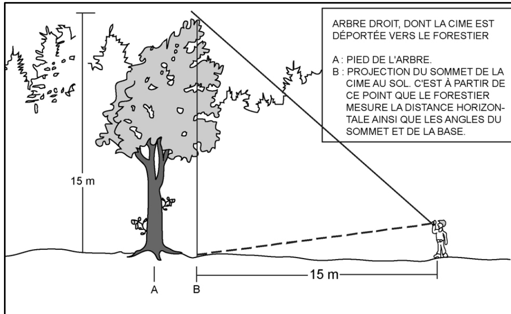
Figure 35 Mesure de hauteur d'arbre (houppier asymétrique)
