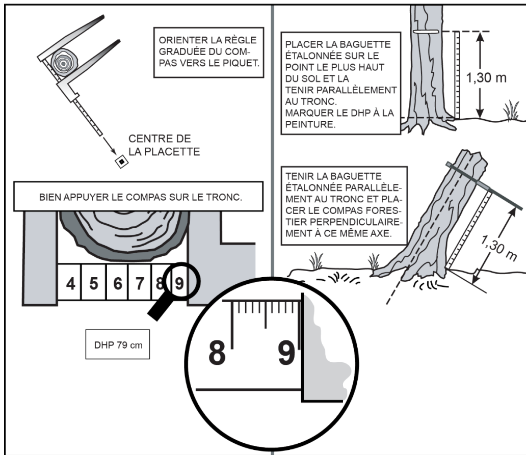
Figure 19 Mesurage du DHP
