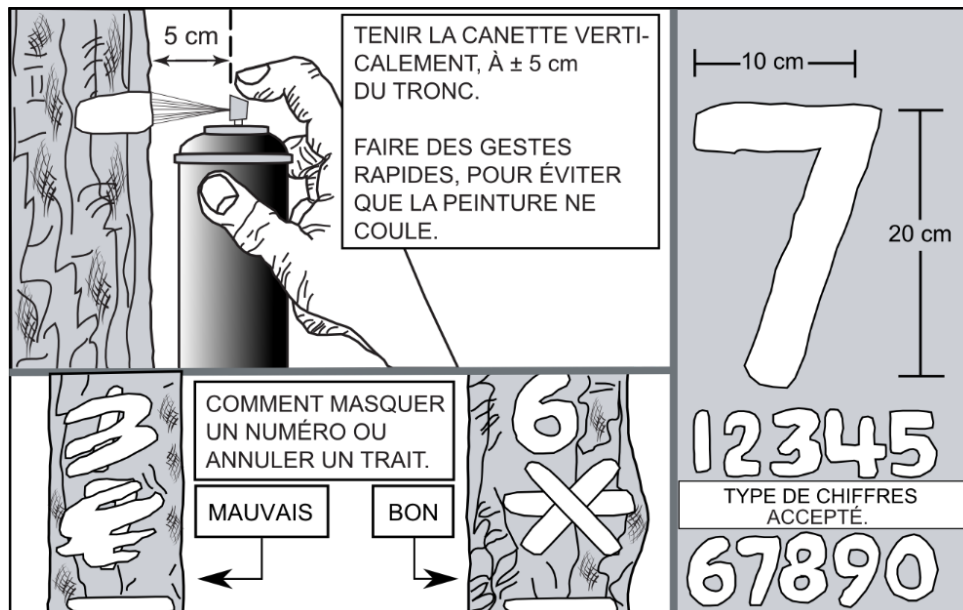
Figure 15 Numérotation de l'arbre à la peinture en aérosol
