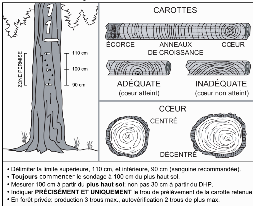
Figure 39 Prélèvement de carottes
