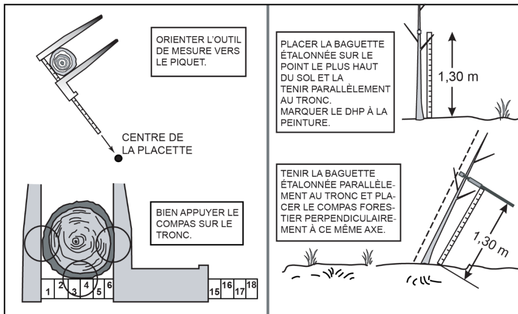
Figure 8 Diamètre à hauteur poitrine (gaules)
